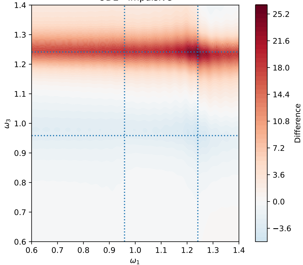
ODE - impulsive
