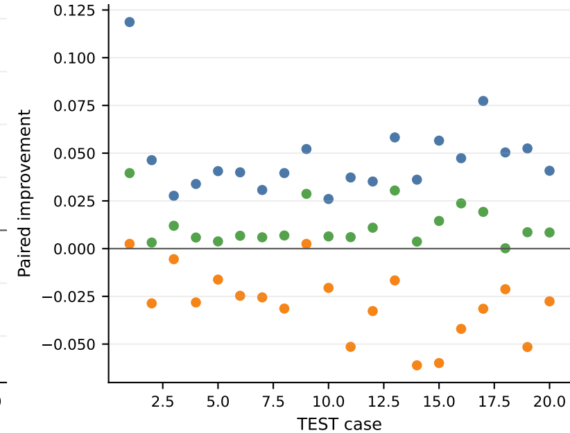
final_wet_iou
