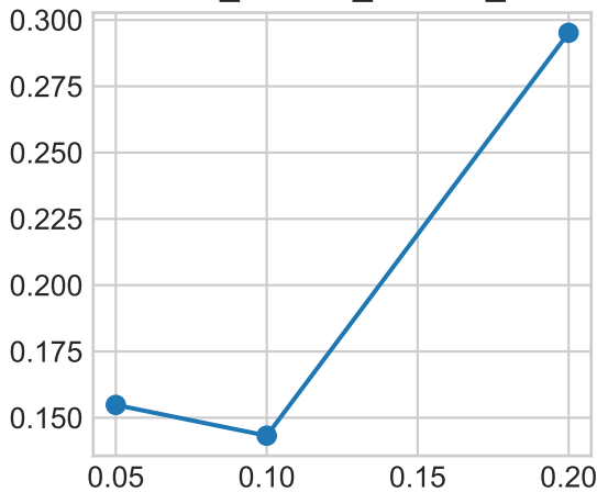
case_validation_time_seconds
