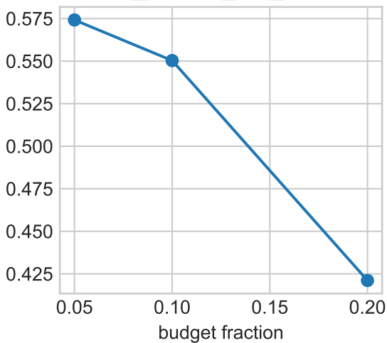
false_positive_fraction
