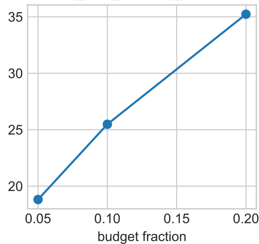
case_validation_time_seconds
