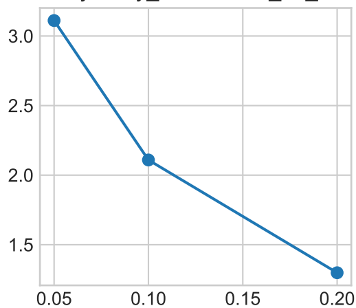
false_positive_fraction
