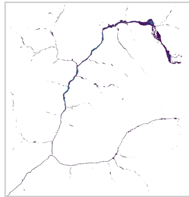
|RiskTemporal-reference|
