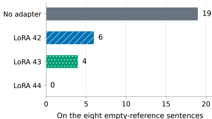
(d) False-positive spans
