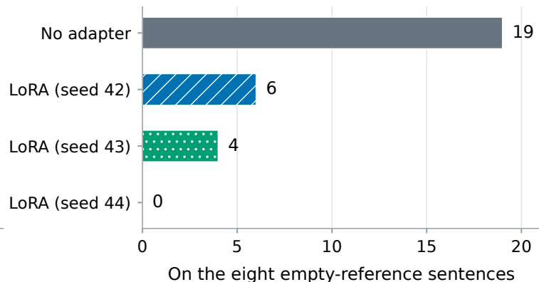
(d) False-positive spans
