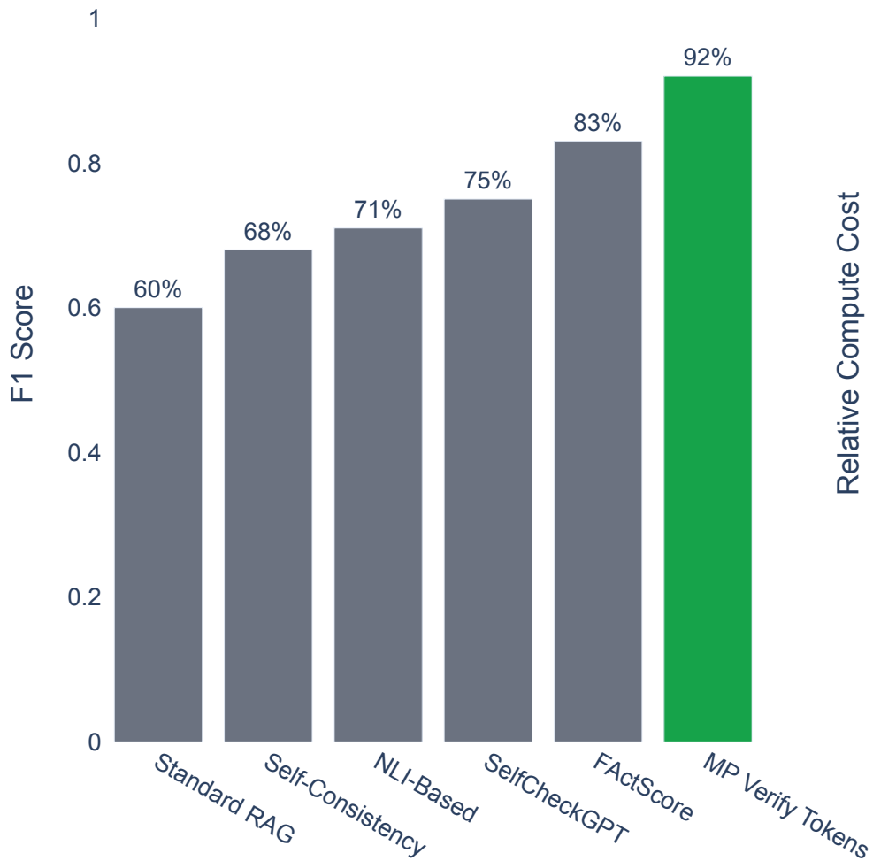
Hallucination Detection F1
