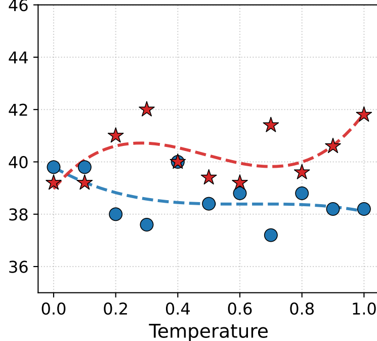
LLaDA-1.5 (MATH)
