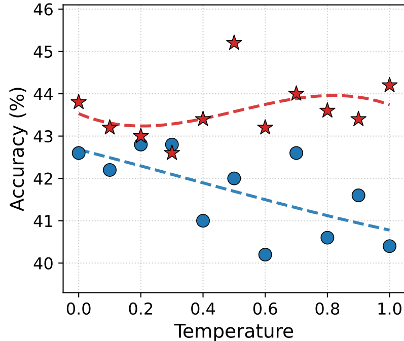
LLaDA-1.5 (MBPP)
