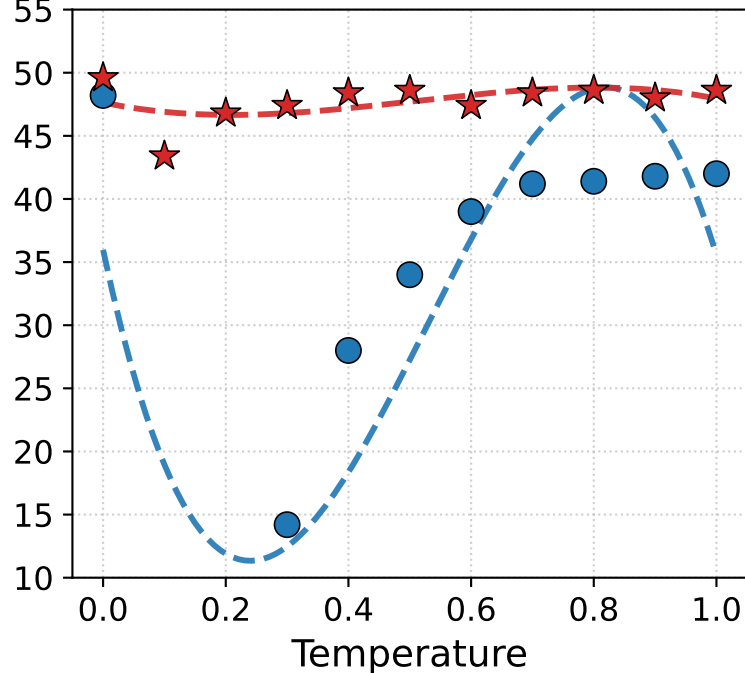
Dream-7B (MBPP)
