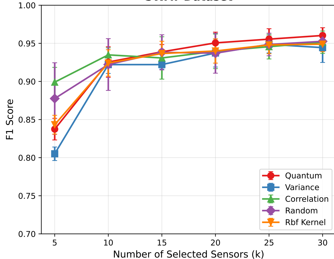
SWAT Dataset
