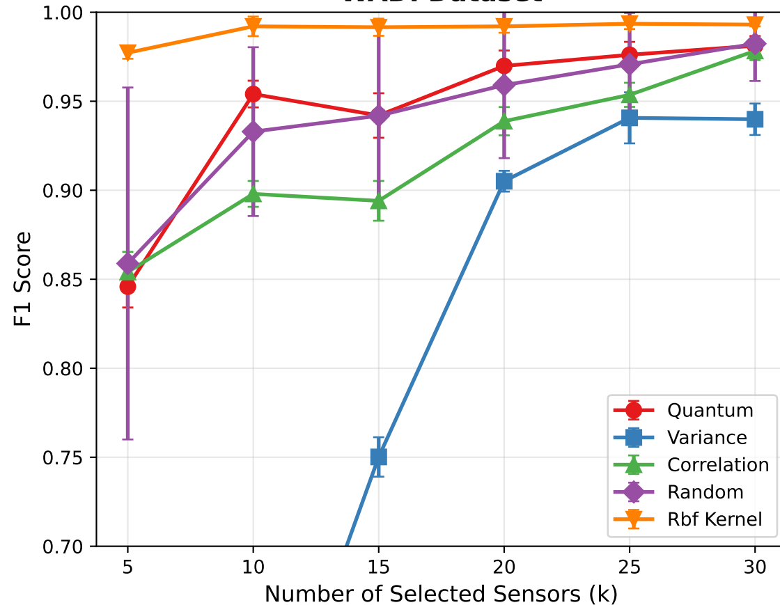
WADI Dataset
