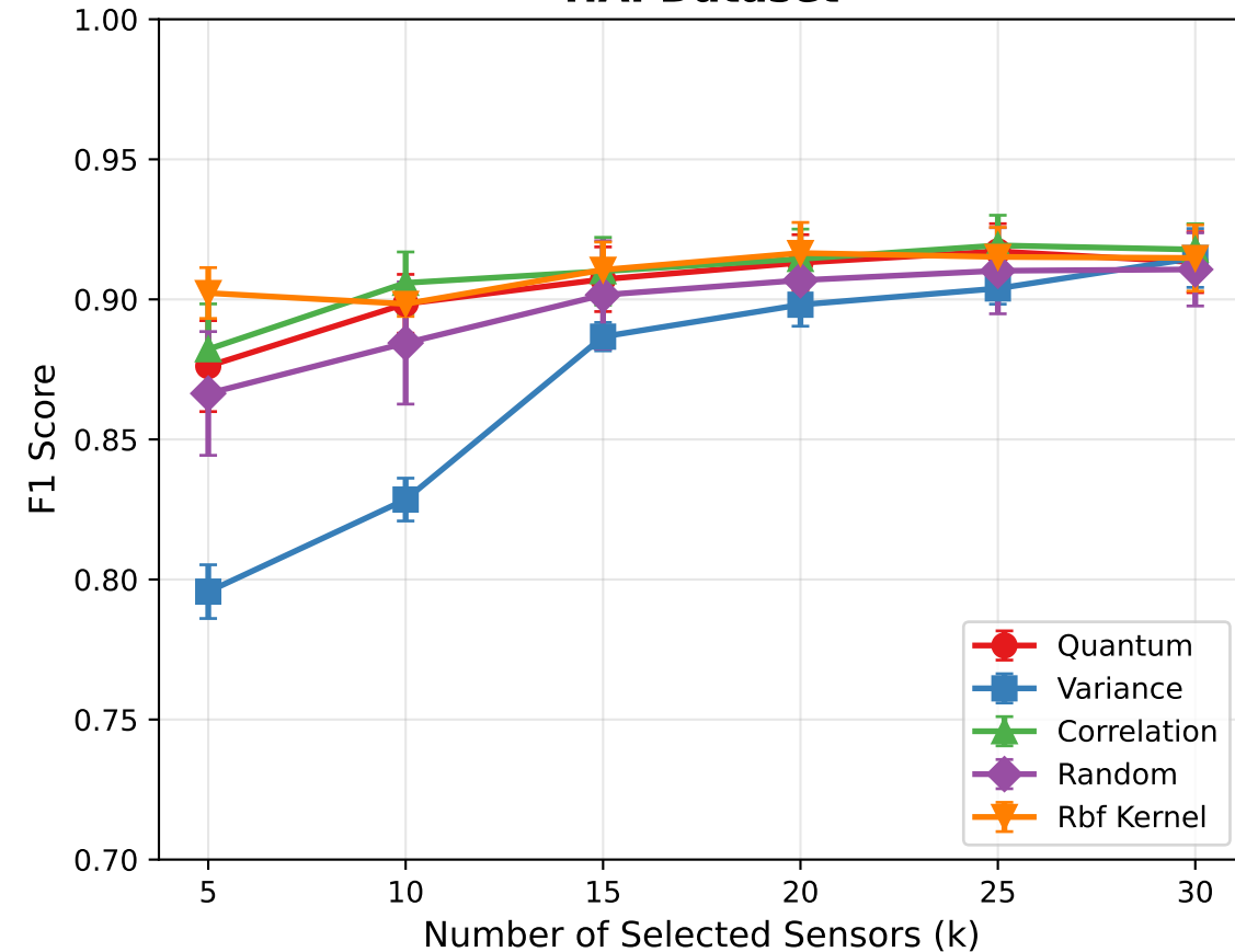
HAI Dataset
