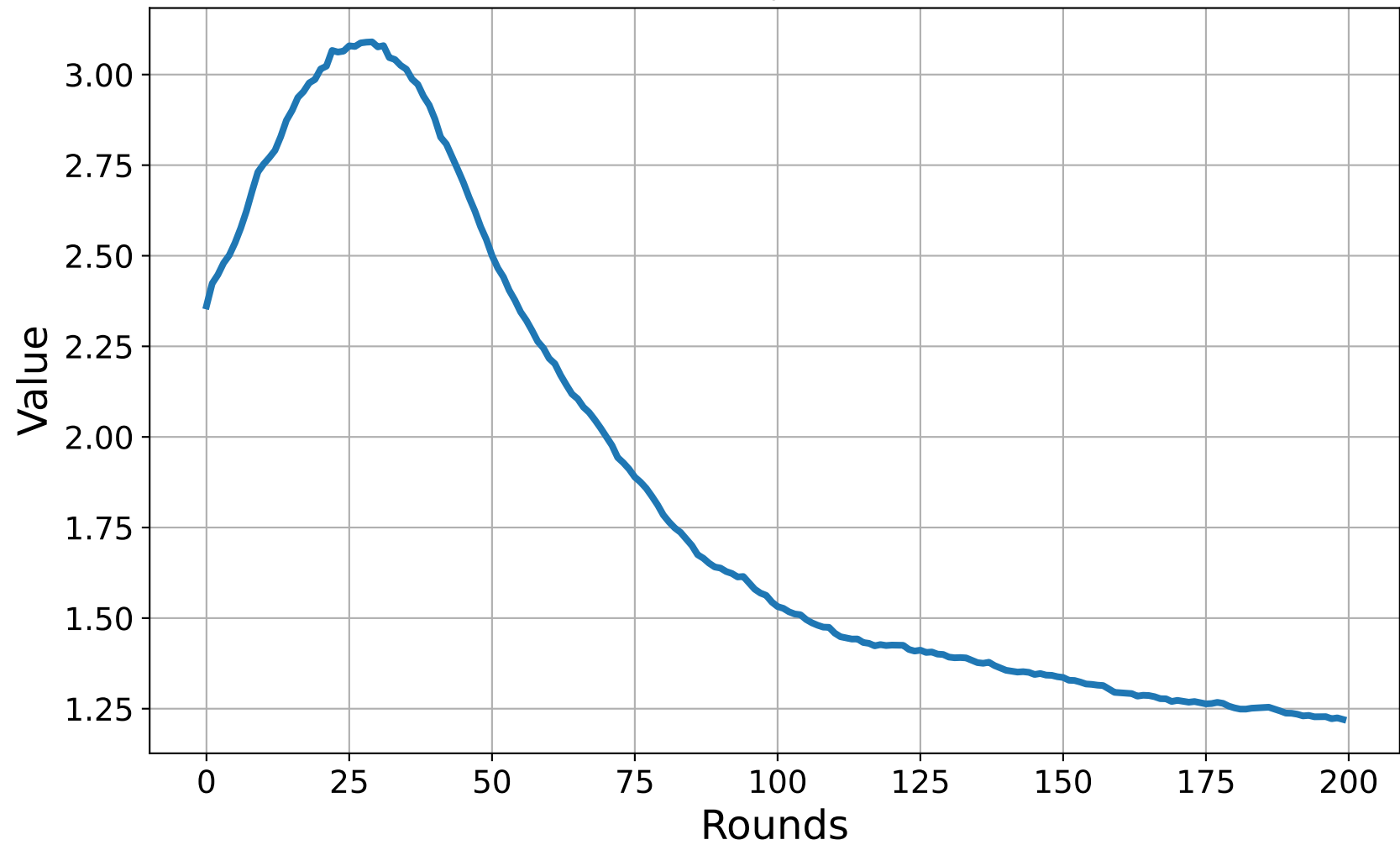
Test Loss per Round
