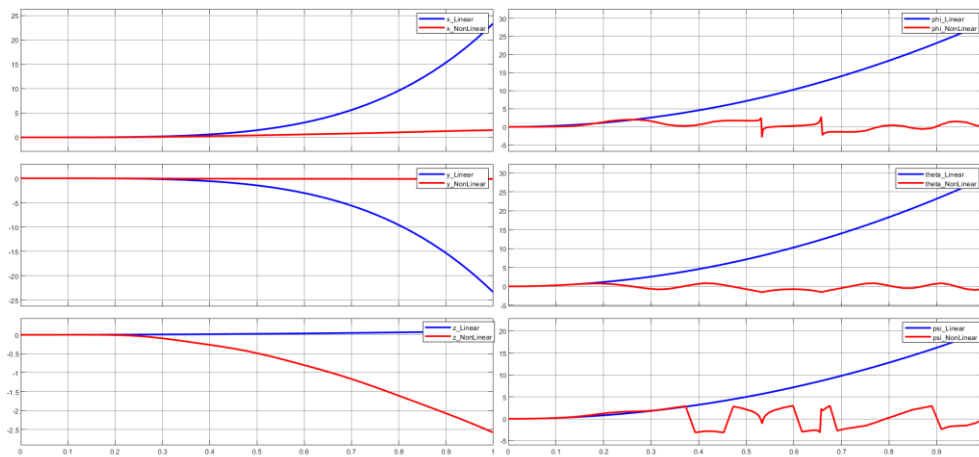
شکل ۲-۳ خروجی سیمولینک برای شرایط اولیه صفر و ورودی ۰.۲
