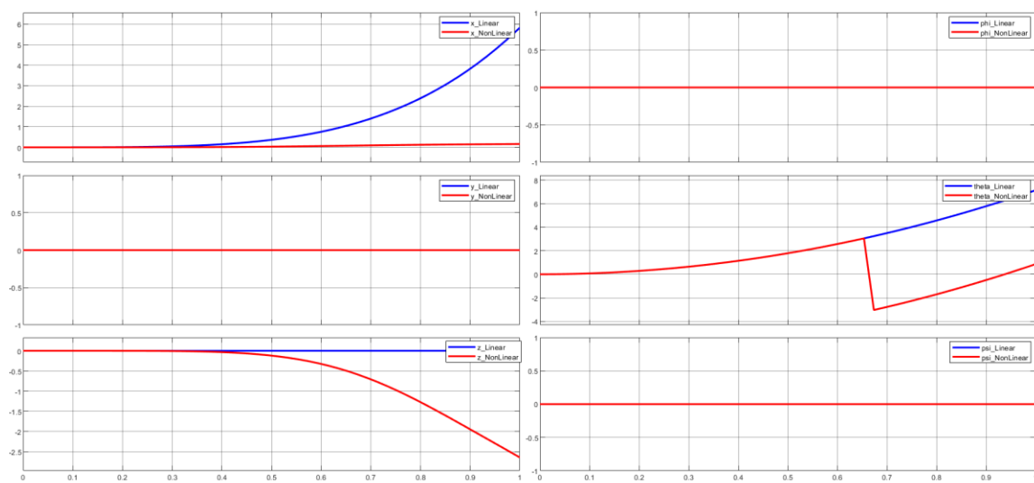
شکل ۵-۳ خروجی سیمولینک برای \delta u_3 = 0.05
