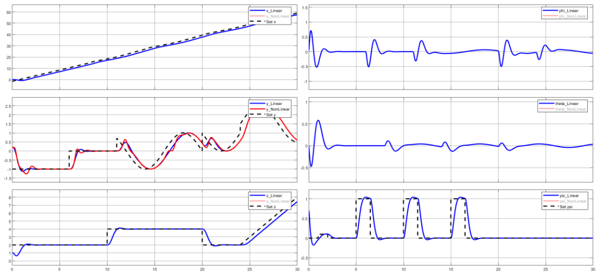
شکل ۴ - ۱ خروجی سیستم تحت کنترل بهینه
