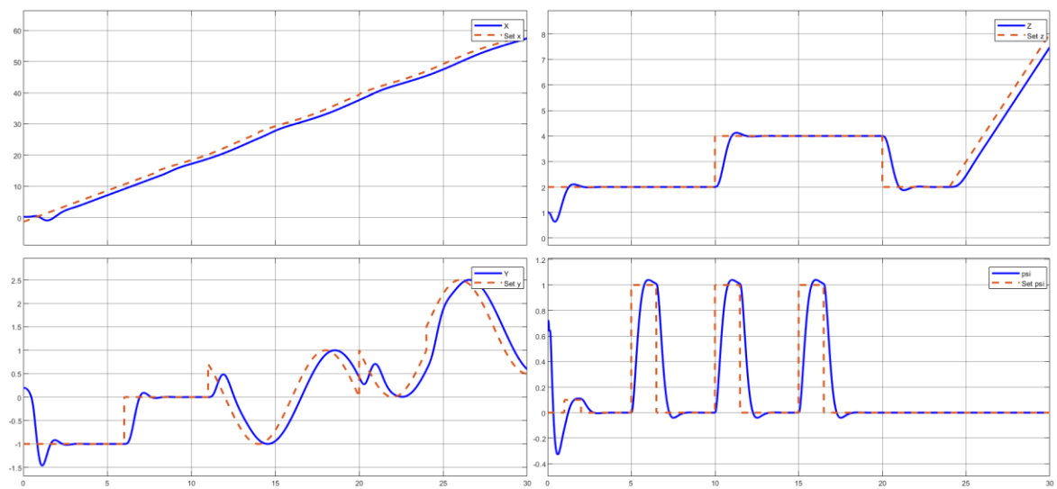
شکل ۴ - ۶ خروجی رویت گر کاهش یافته
