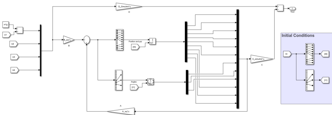
شکل ۳-۷ حالت خطی با انتگرال گیر
