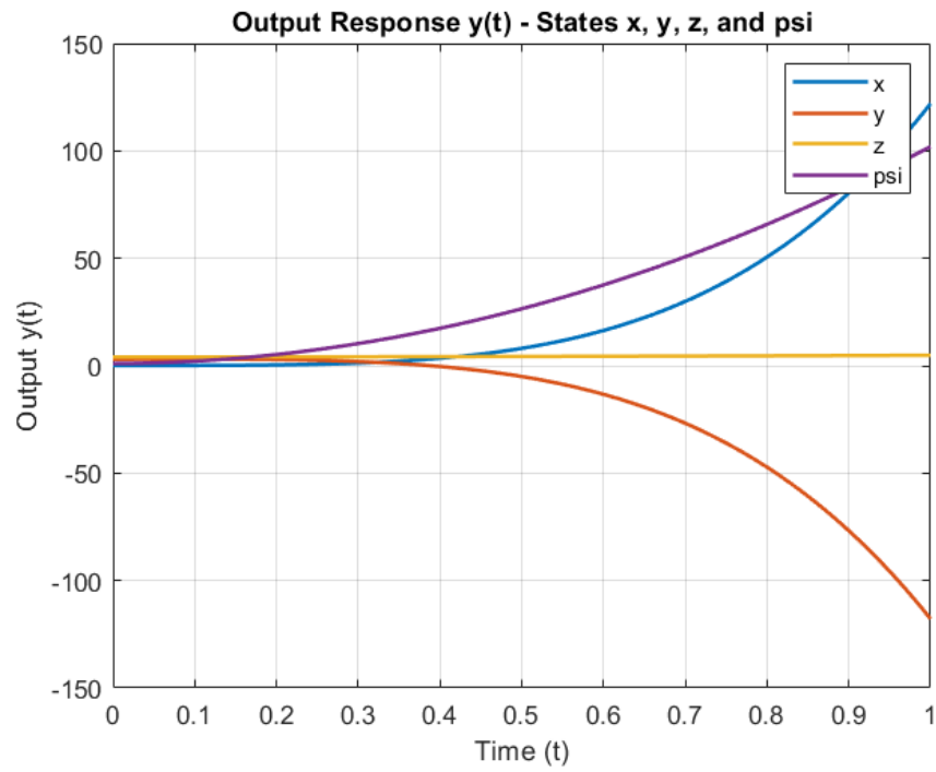
شکل ۱۲-۳ پاسخ خروجی سیستم به شرط اولیه دلخواه و ورودی پله واحد
