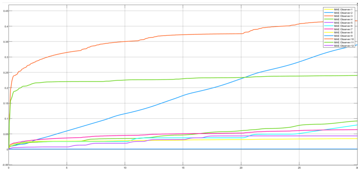
شکل ۴ - ۱۲ MAE رویت گر مرتبه کامل (A1.2)
