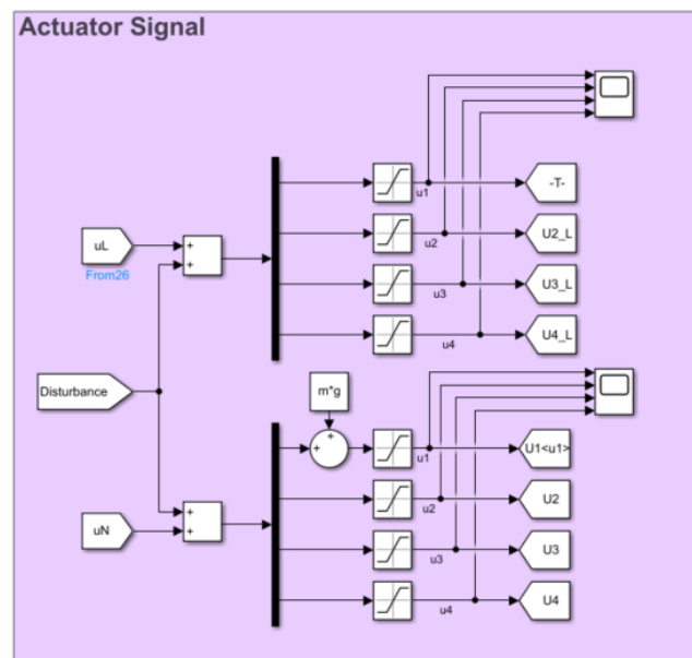
شکل ۴ - ۲ بلوک عملگرها
