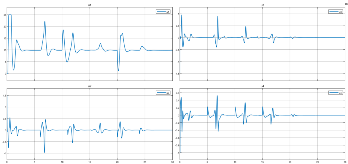
شکل ۴ - ۳ خروجی سیستم تحت کنترل بهینه
