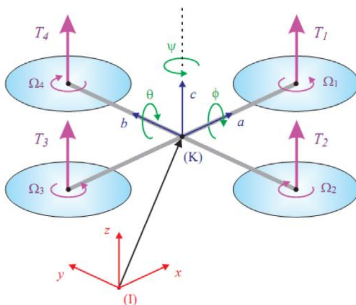
شکل ۱-۲ سیستم کوادروتور ۶ درجه آزادی
