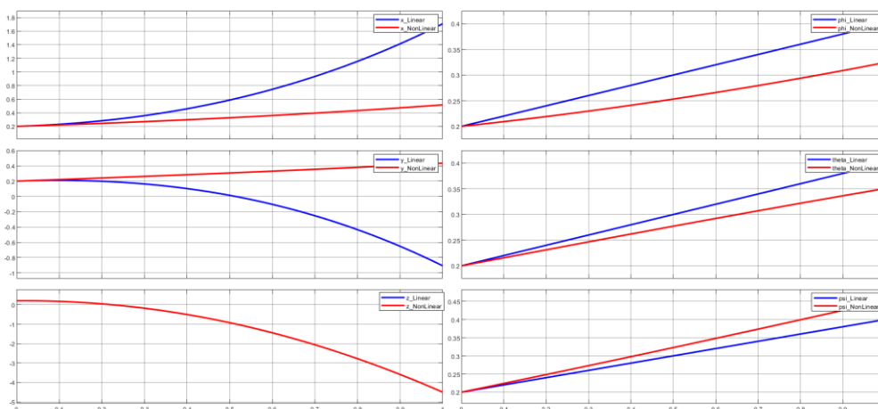
شکل ۳-۱ خروجی سیمولینک برای شرایط اولیه یک و ورودی صفر
