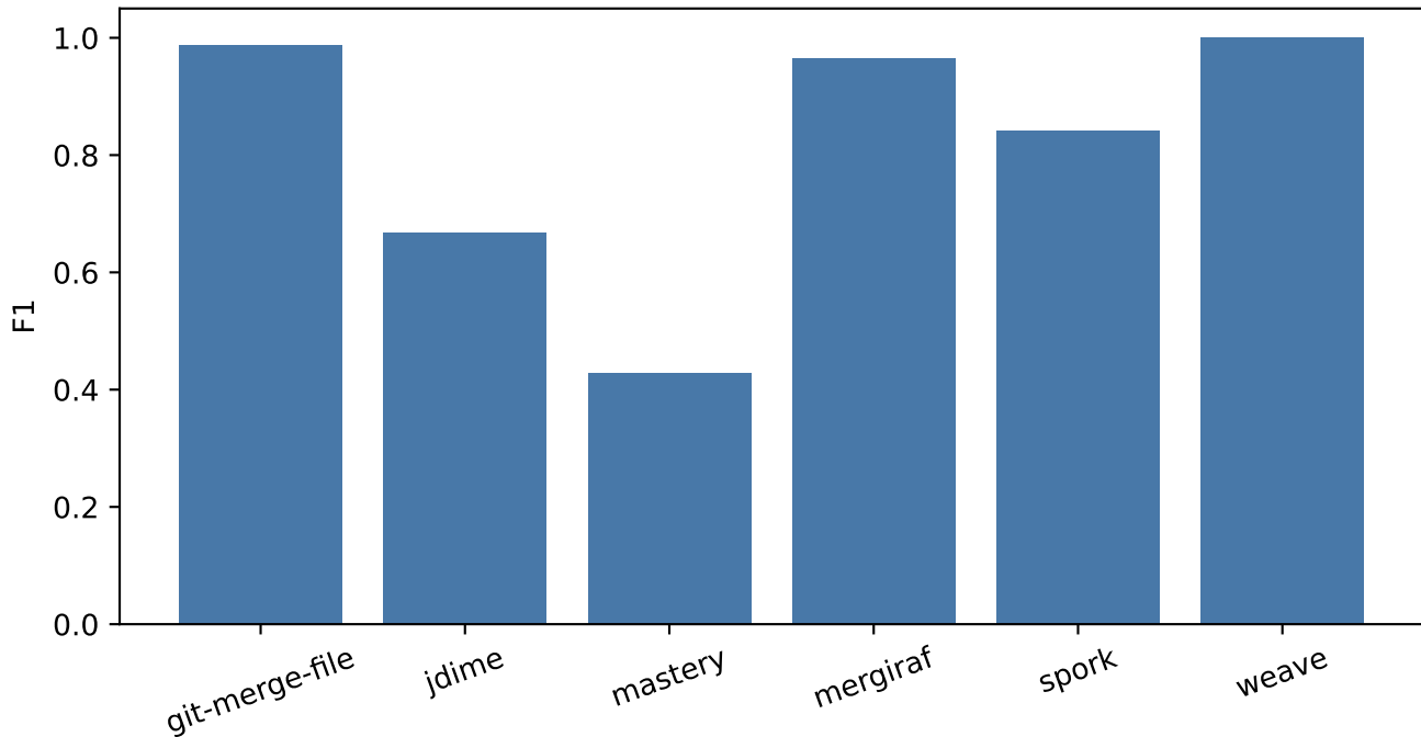
F1 per tool (n=50 scenarios)
