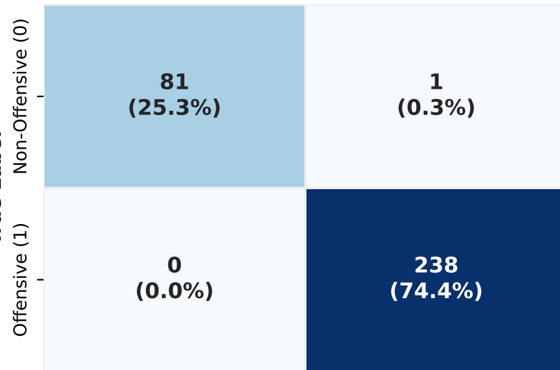
(d) CNN-BiLSTM [Deep Learning] Macro-F1: 0.9959
