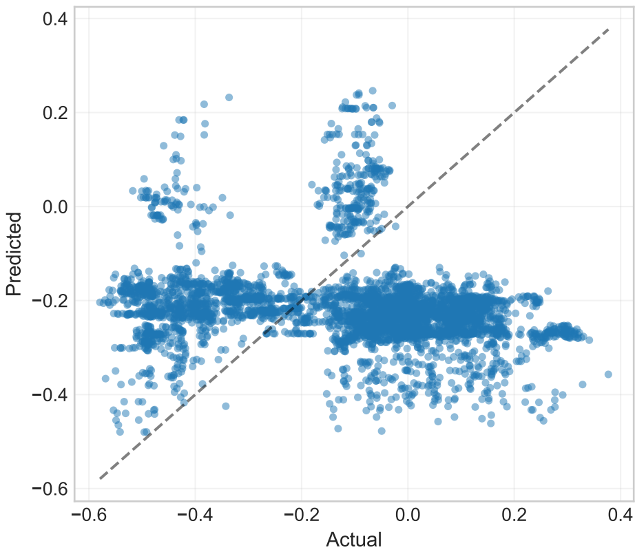
fusion
