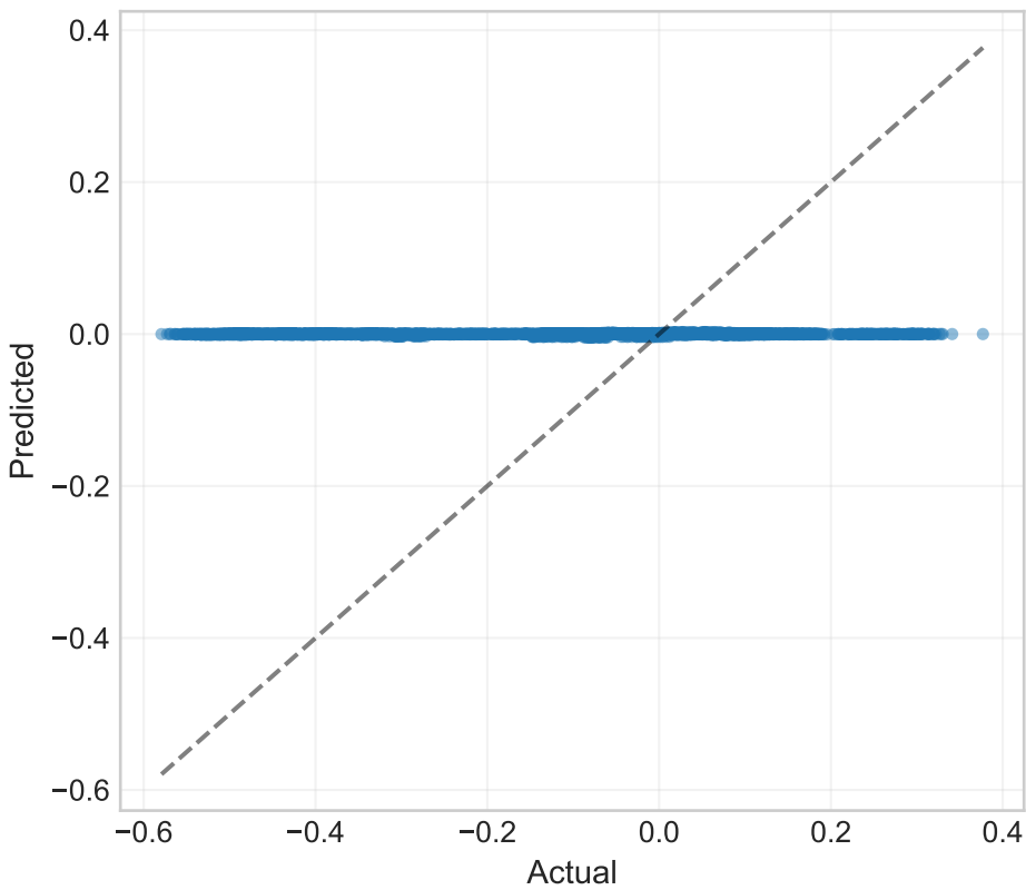
fusion
