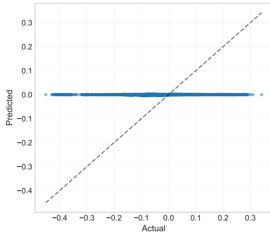
fusion
