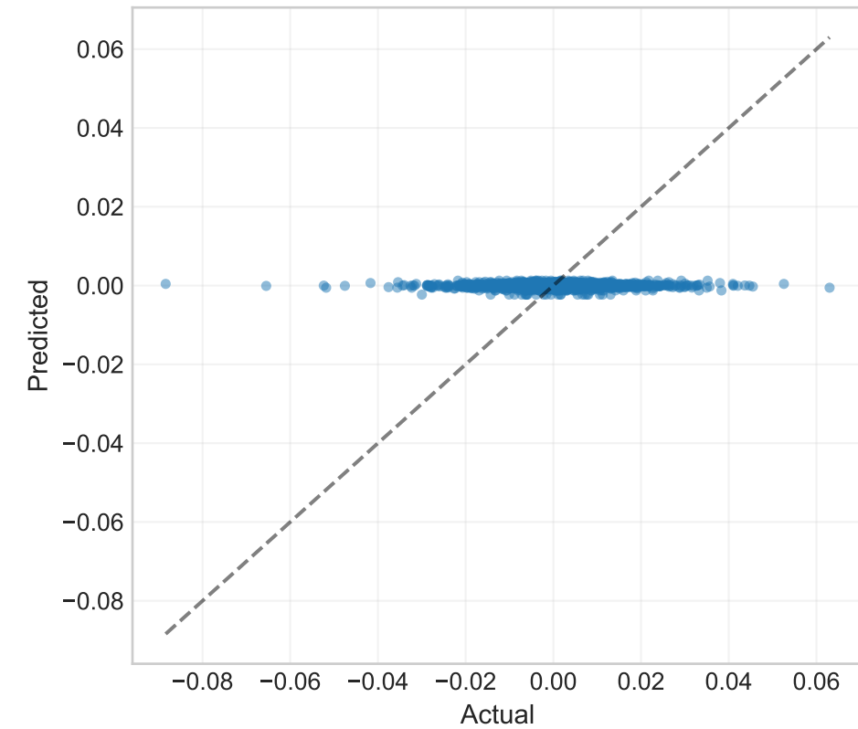
fusion
