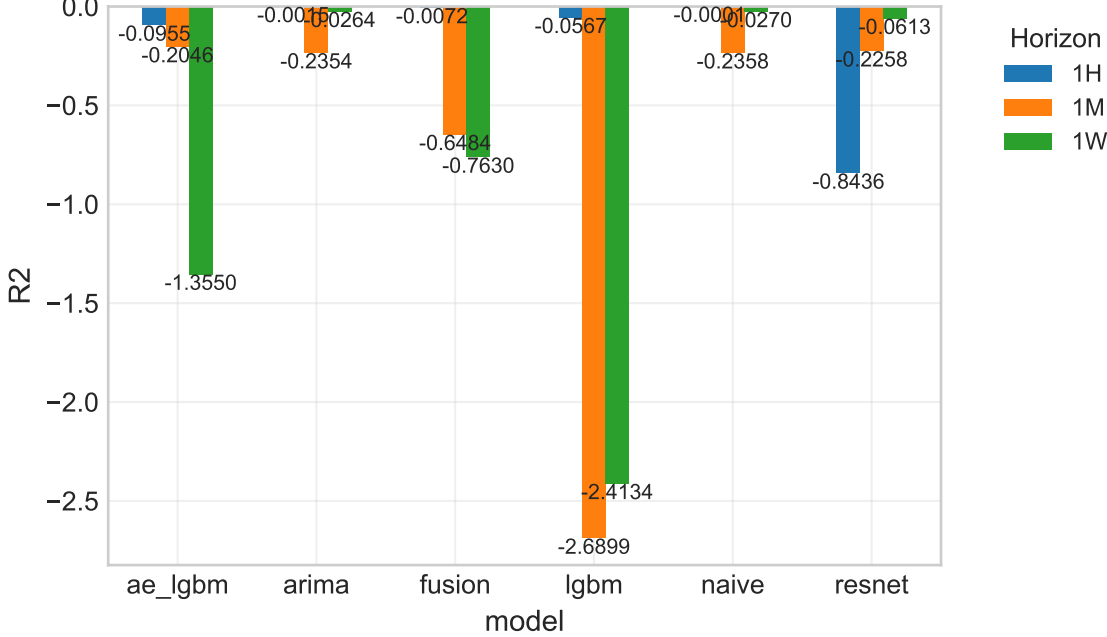
R2
