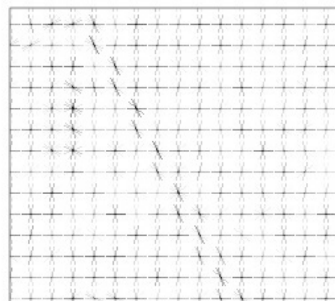
Sobel HOG
