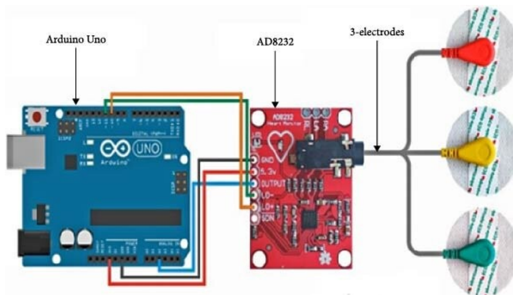
و سه الکترود AD8232 مازول، Arduino Uno شکل پیوست-۲: اتصال
