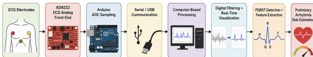
شکل ۱-۳ - ساختار کلی سامانه پیشنهادی پایش بلادرنگ ECG
