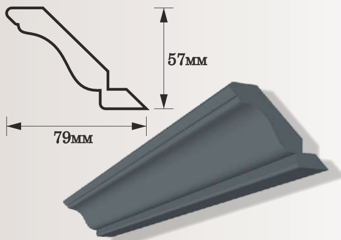
Карниз №118 Семачка
