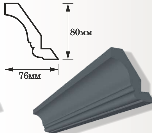
Карниз №123
