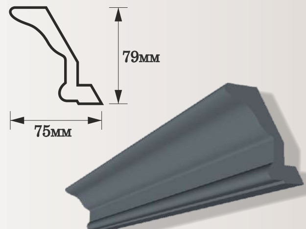
Карниз №124 Шашки
