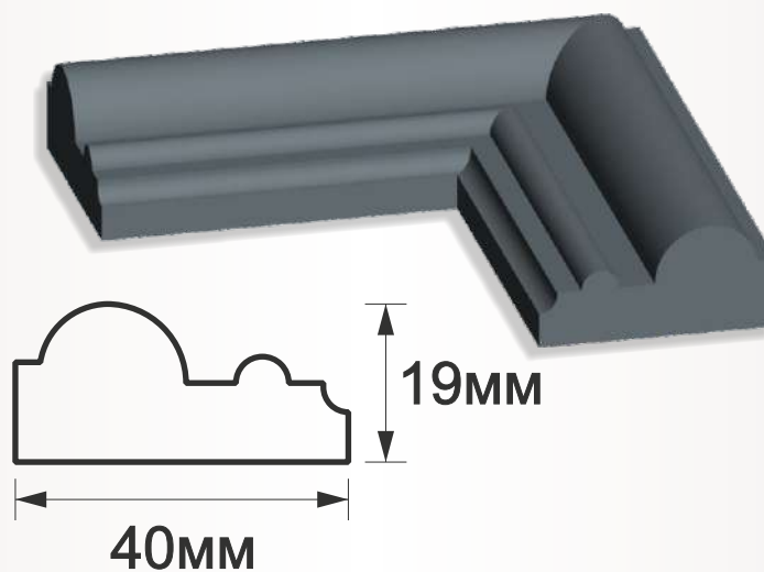
Штапик 2
