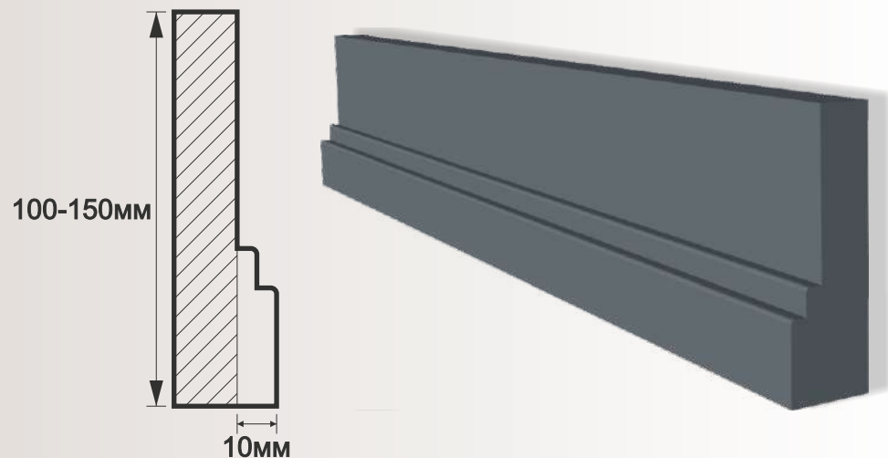
Цоколь с сапожком
