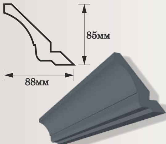
Карниз №118 Семачка
