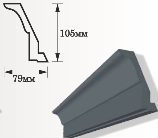
Карниз №123
