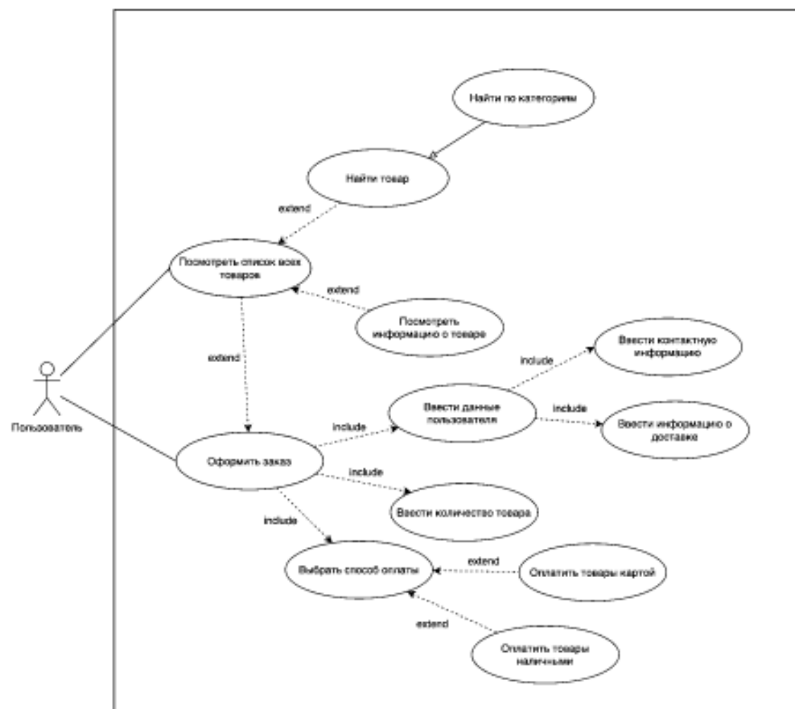
Рисунок 2. Диаграмма Use Case для версии 2.0 веб-приложения «Накарабине»
