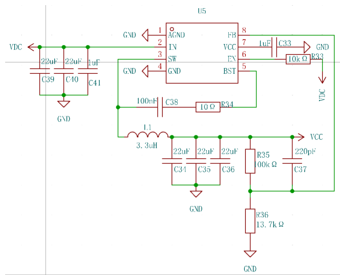
图2 MP2236模块
