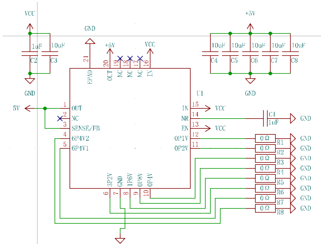
图1 TPS7A47模块
