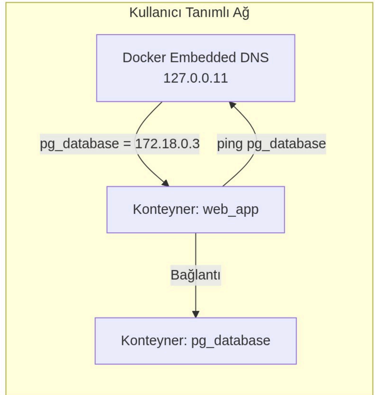
Şekil: Docker Embedded DNS Çalışma Mantığı
