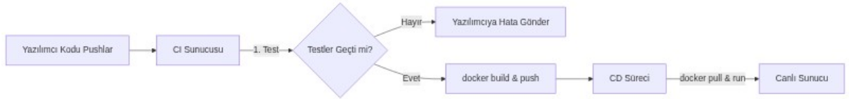
Şekil: Docker Tabanlı CI/CD Boru Hattı (Pipeline)
