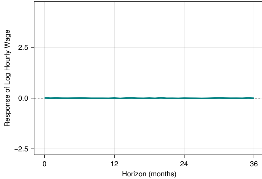
(8) Precision_prod_repair
