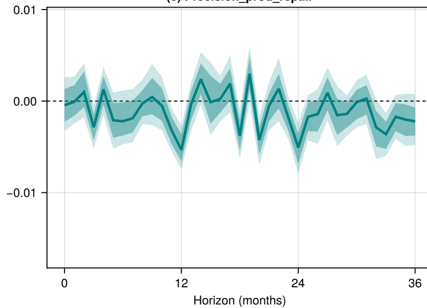
(8) Precision_prod_repair
