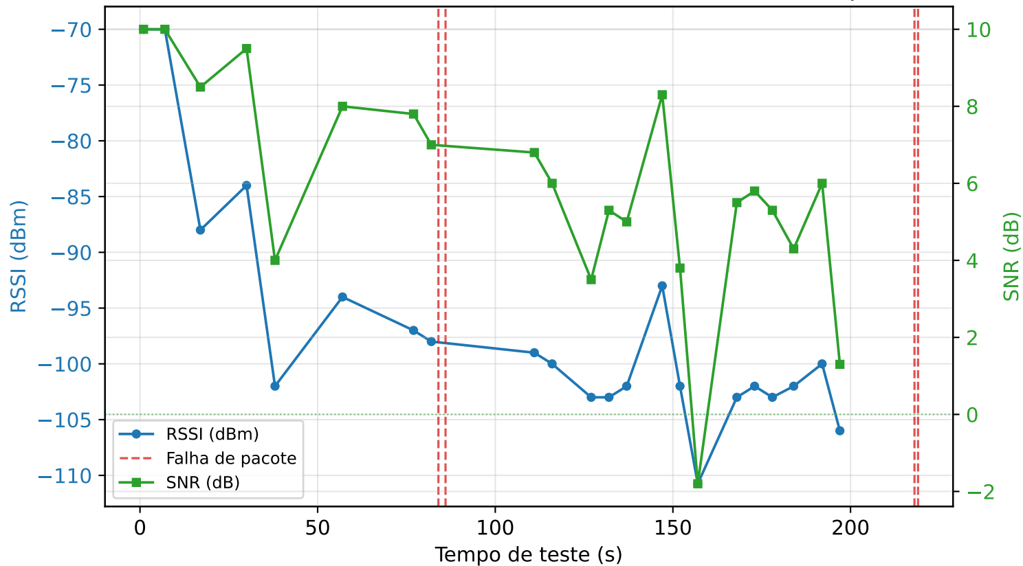
Estabilidade do Enlace Durante Teste Dinâmico de Campo
