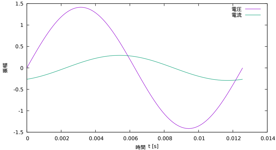
LC共振回路の電圧・電流波形
