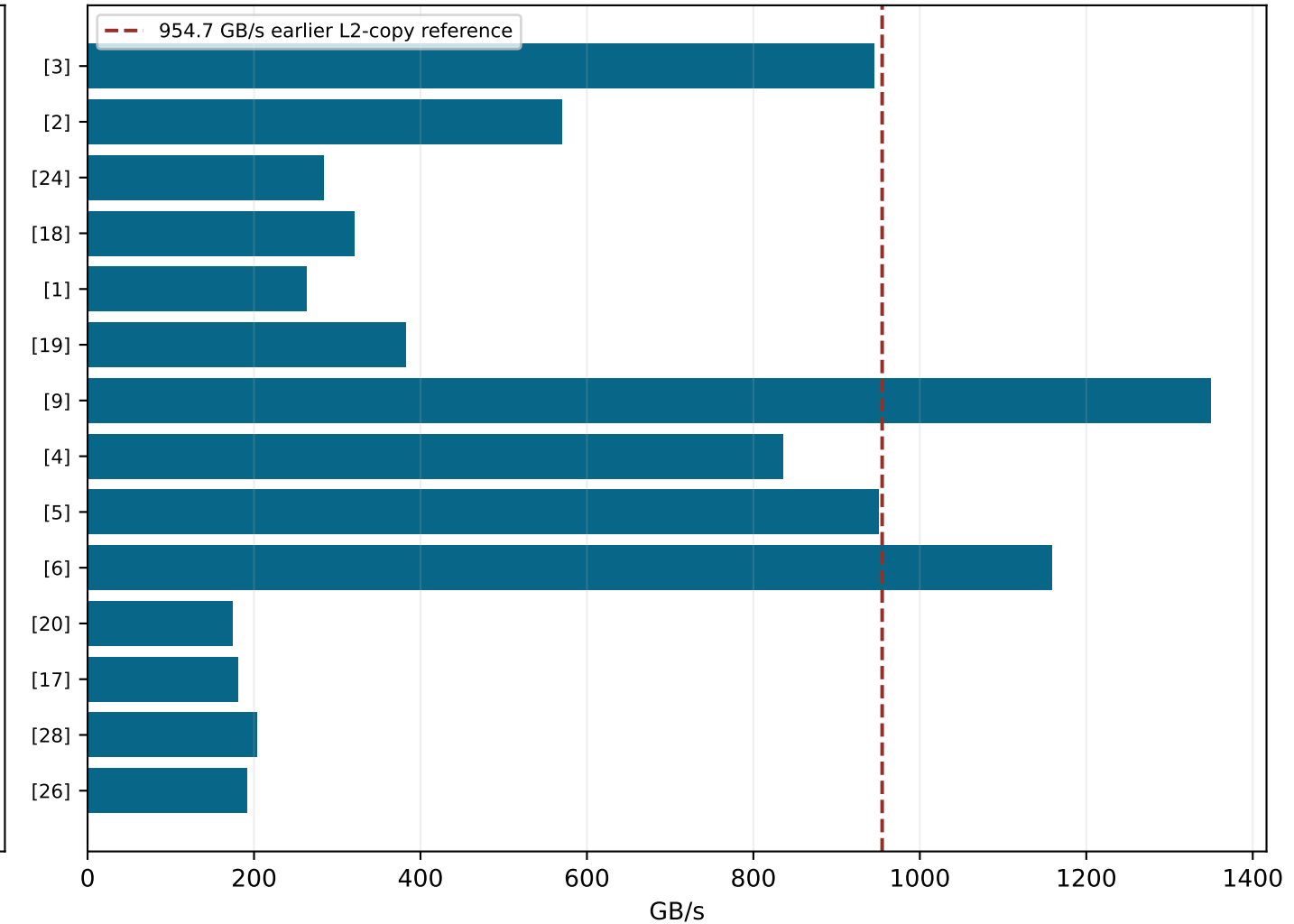
Actual L2 byte counter / NCU kernel time
