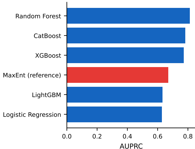
(a) Precision-recall AUC
