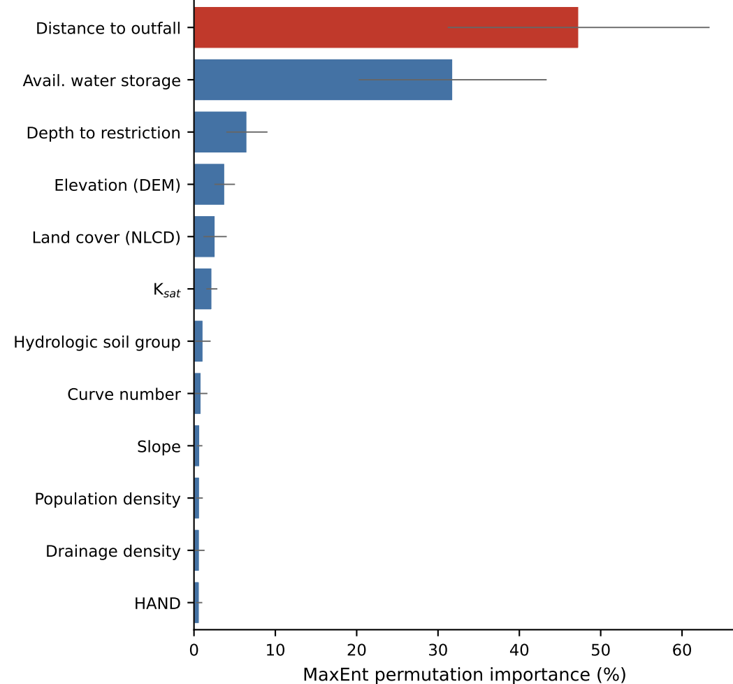
(a) MaxEnt permutation importance
