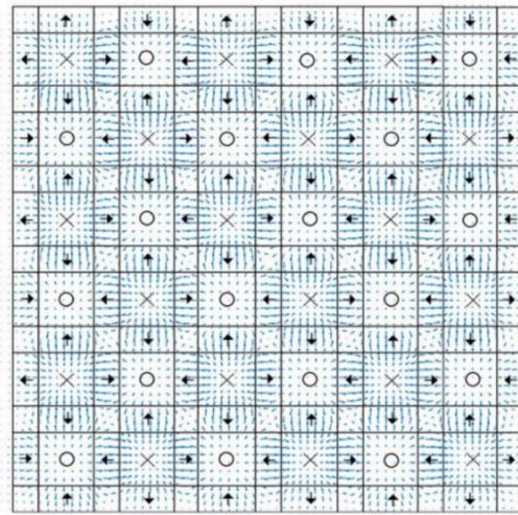
(آ) آرایه هالباخ دوبعدی و میدان مغناطیسی آن [۱۸] (ب) آرایه هالباخ دوبعدی با قطعات آهنی در فضاهای خالی [۹]
