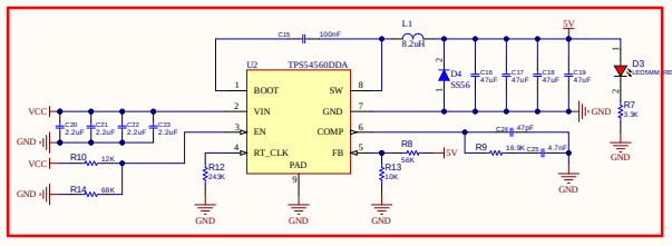
Adaptor 9V~24V
