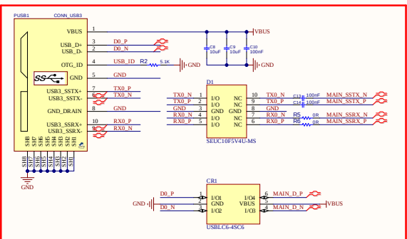
Input USB3.0
