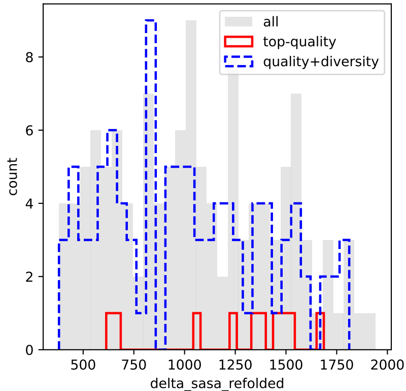
delta_sasa_refolded
