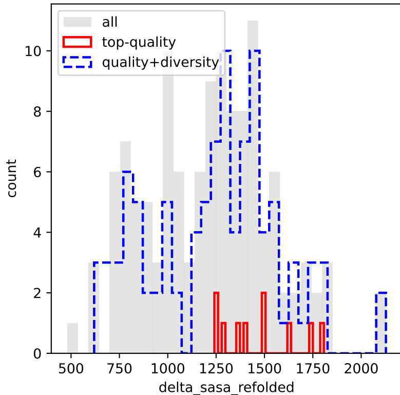
delta_sasa_refolded
