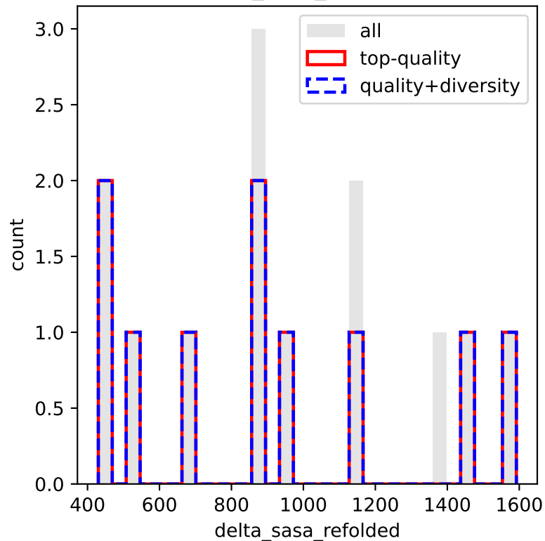
delta_sasa_refolded
