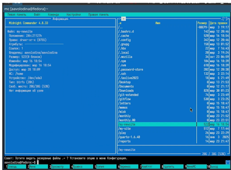
Рисунок 5.8: информация о каталоге
