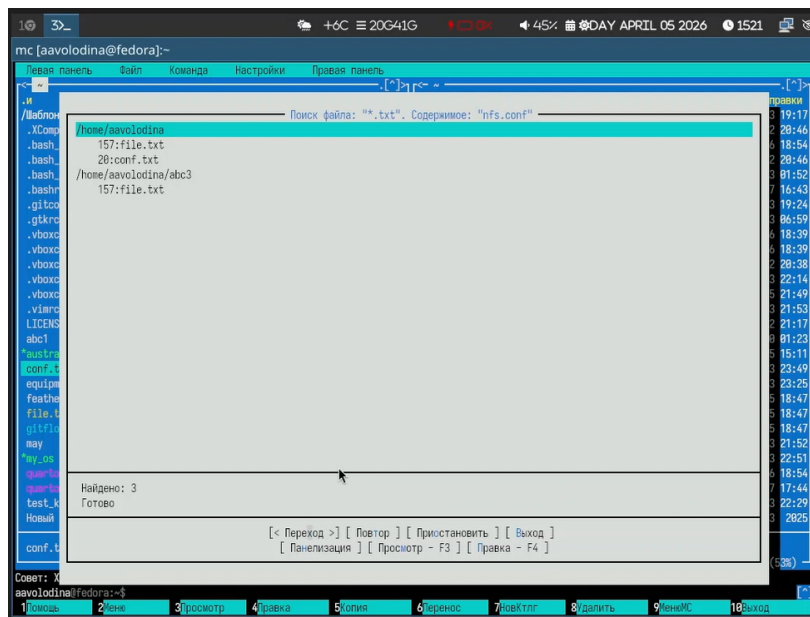
Рисунок 5.18: поиск с учетом фильтров
