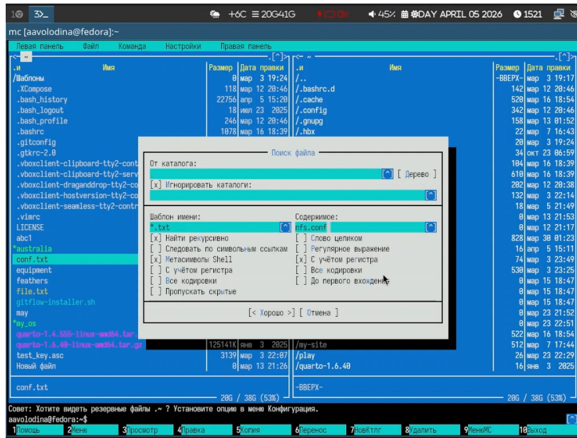
Рисунок 5.17: поиск с учетом фильтров
