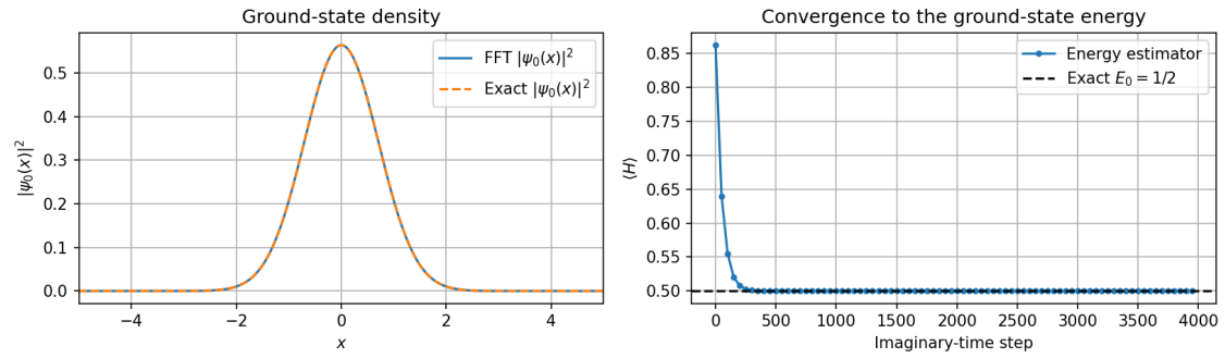
Figura 9: Estado fundamental del oscilador armónico cuántico obtenido mediante propagación en tiempo imaginario con el método split-operator basado en FFT. Izquierda: densidad de probabilidad |\psi_0(x)|^2 numérica frente a la gaussiana analítica \pi^{-1/2}e^{-x^2} . Derecha: convergencia del estimador de energía \langle H \rangle al valor exacto E_0 = 1/2 .
