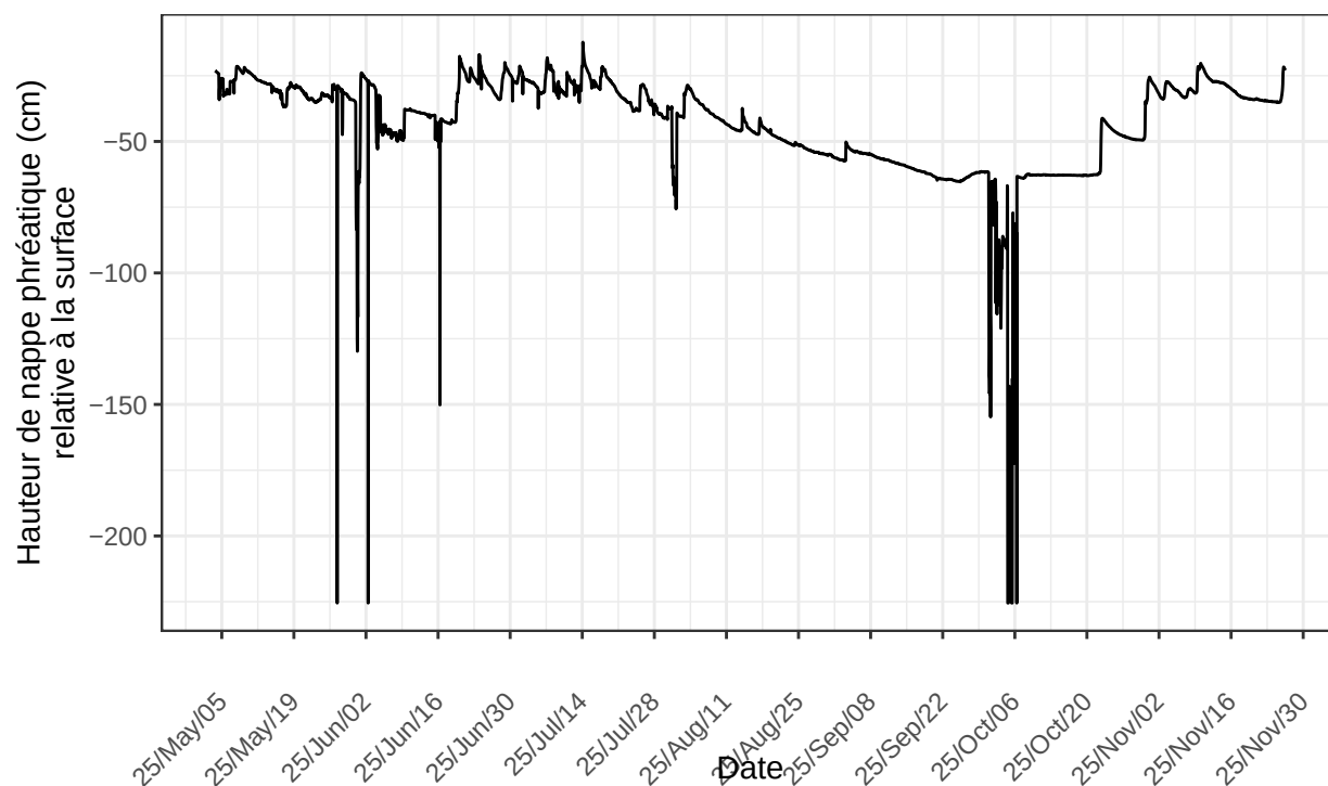
St-Henri, sonde no 42563 à l'emplacement STH.C.p9m.2025 nombre de ligne du fichier : 4988
