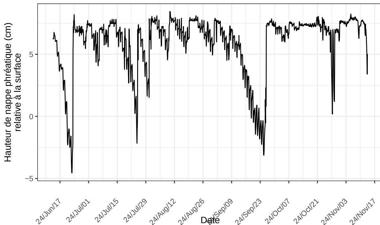
St-Henri, sonde no 41359 à l'emplacement STH.D2.p8m.2025 nombre de ligne du fichier : 4985
