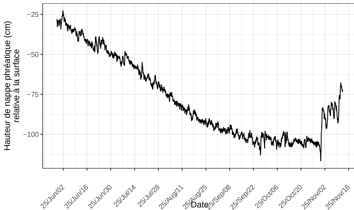
Inkerman, sonde no 22224394 à l'emplacement INK.pasMare.D1.p30m.2025 nombre de ligne du fichier : 4036
