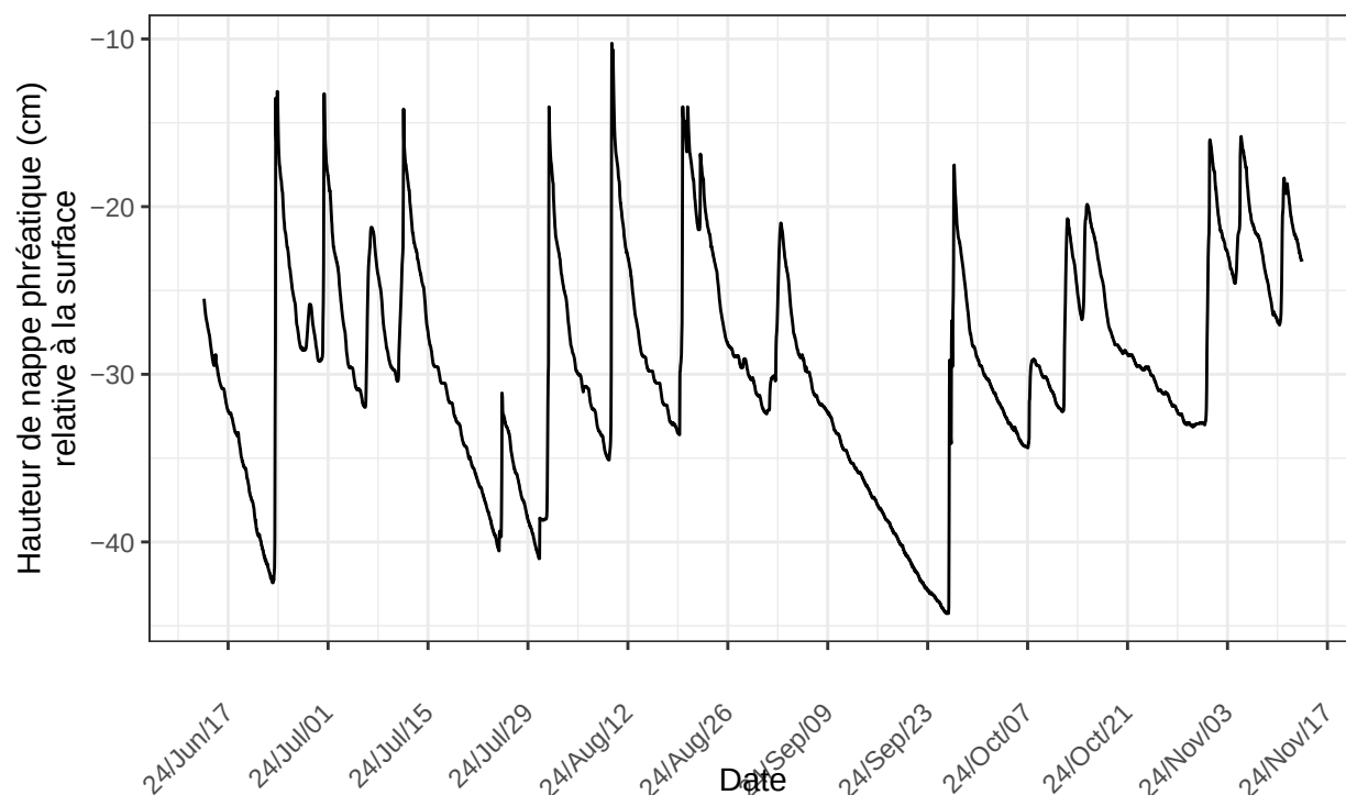
St-Henri, sonde no 42565 à l'emplacement STH.C.p6m.2025 nombre de ligne du fichier : 4988
