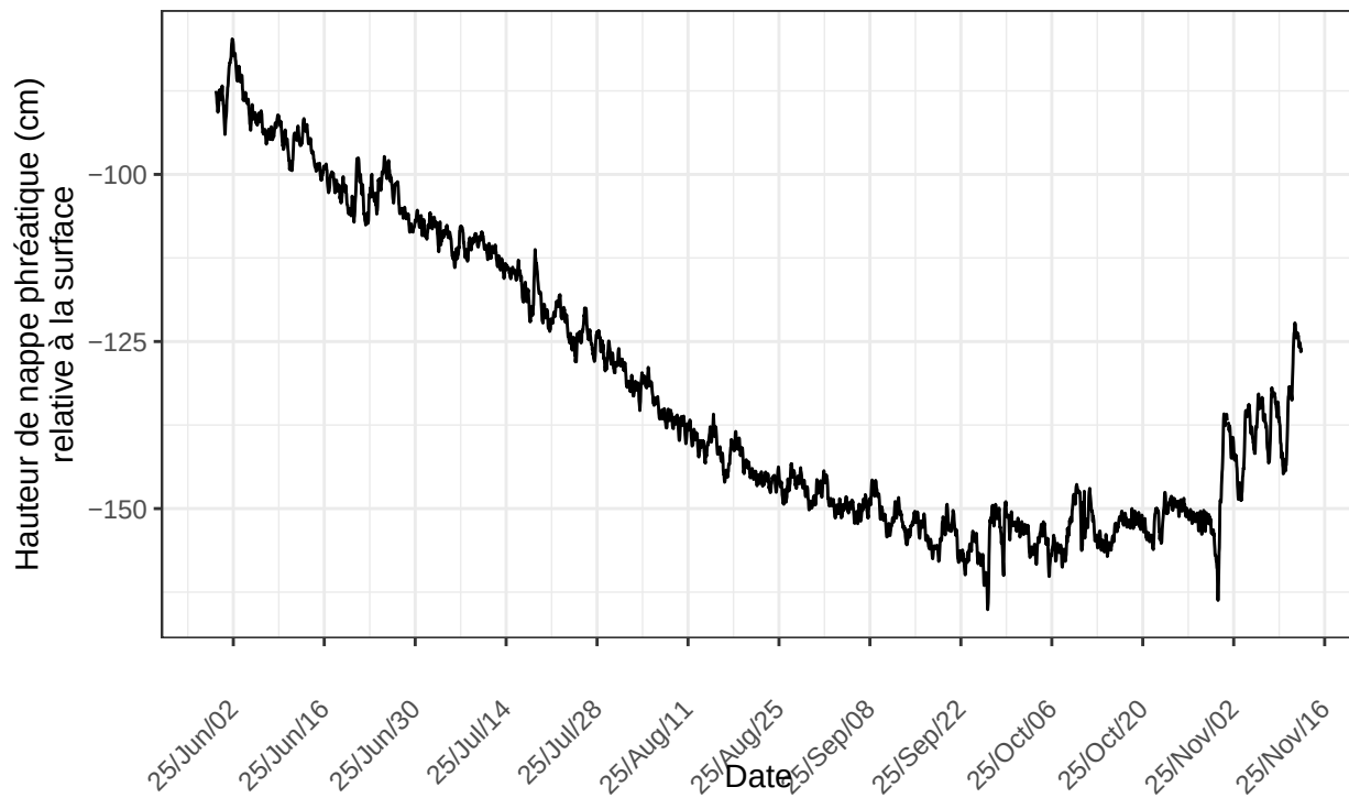
Inkerman", sonde no 22224388 à l'emplacement INK.pasMare.A1.p7m.2025 nombre de ligne du fichier : 4011
