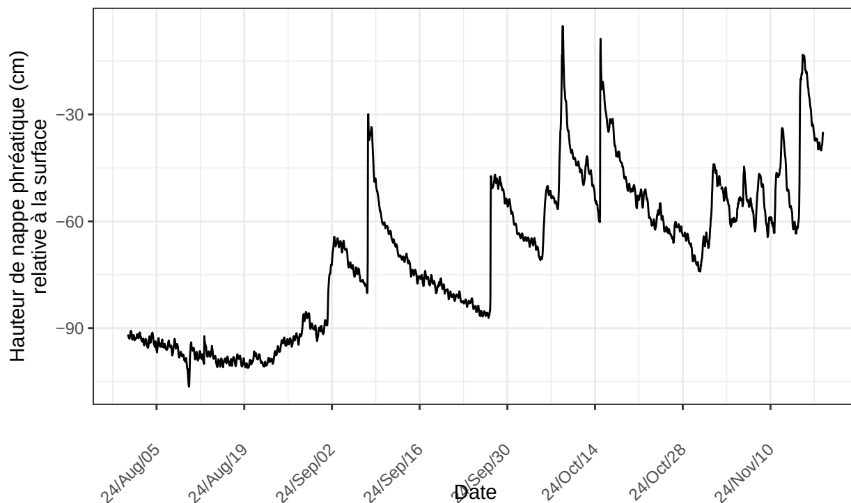
Inkerman, sonde no 20853328 à l'emplacement INK.EA.m4m.2024 nombre de ligne du fichier : 3148
