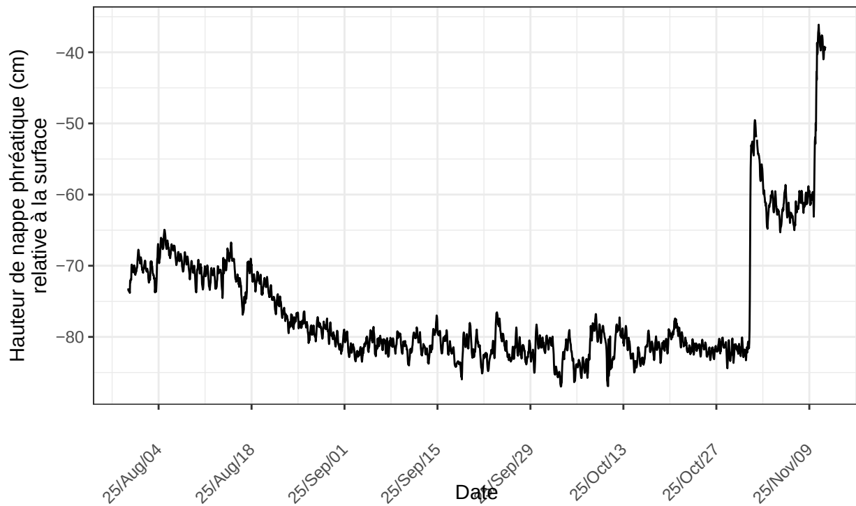
Inkerman", sonde no 22224414 à l'emplacement INK.pasMare.C2.p30m.2025 nombre de ligne du fichier : 4035
