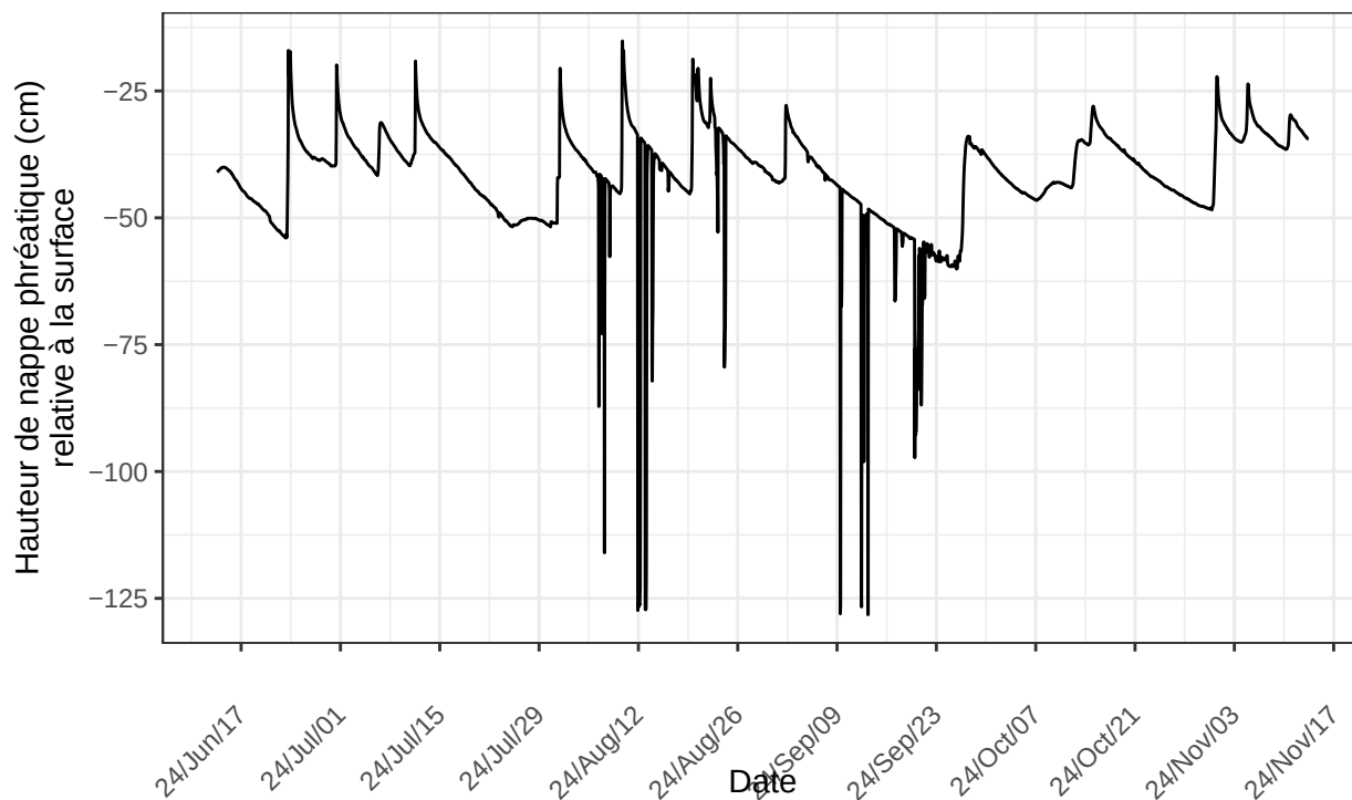
St-Henri, sonde no 41362 à l'emplacement STH.D3.10m.2024 nombre de ligne du fichier : 3692
