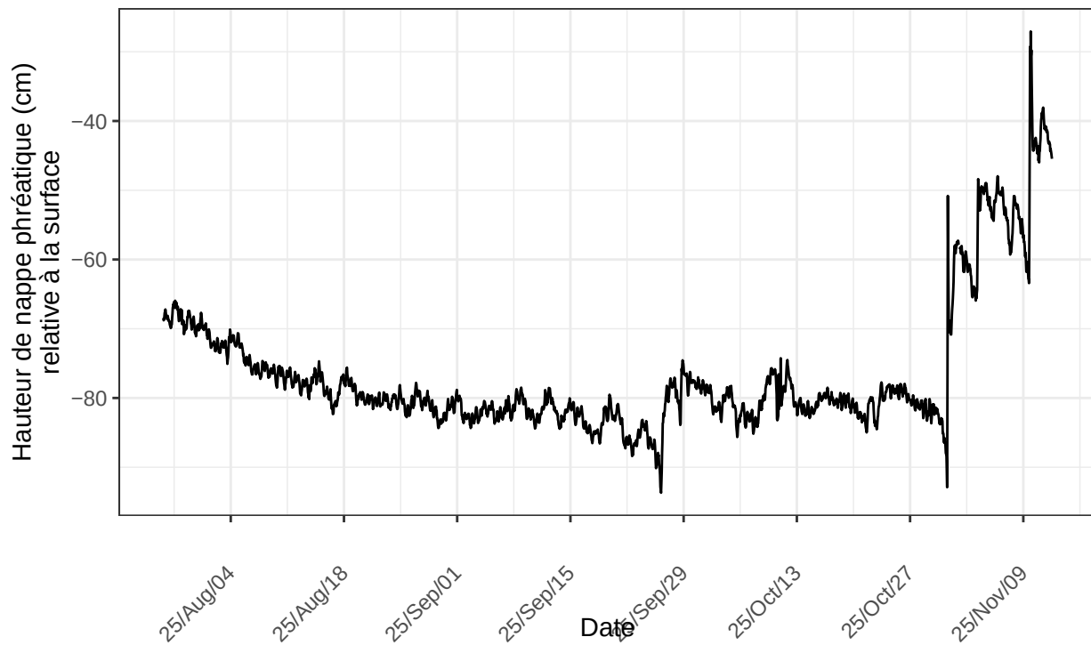
Président-Ouest", sonde no 22220781 à l'emplacement PRO.ch1.R23.2025 nombre de ligne du fichier : 4556
