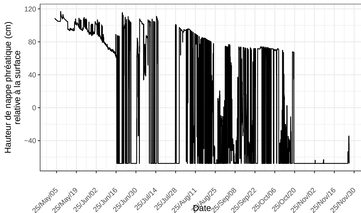
St-Henri, sonde no 42565 à l'emplacement STH.C.p6m.2025 nombre de ligne du fichier : 4988
