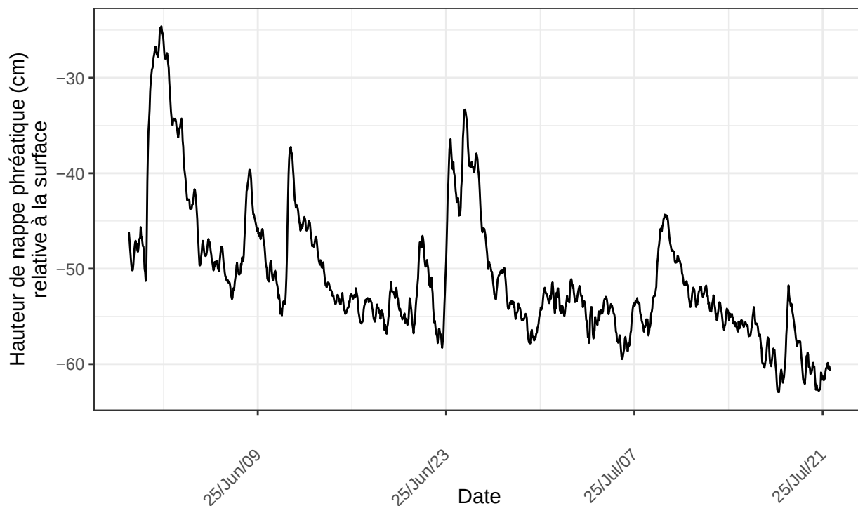
Président-Ouest, sonde no 22224386 à l'emplacement PRO.ch1.T1.gr.protec nombre de ligne du fichier : 1293
