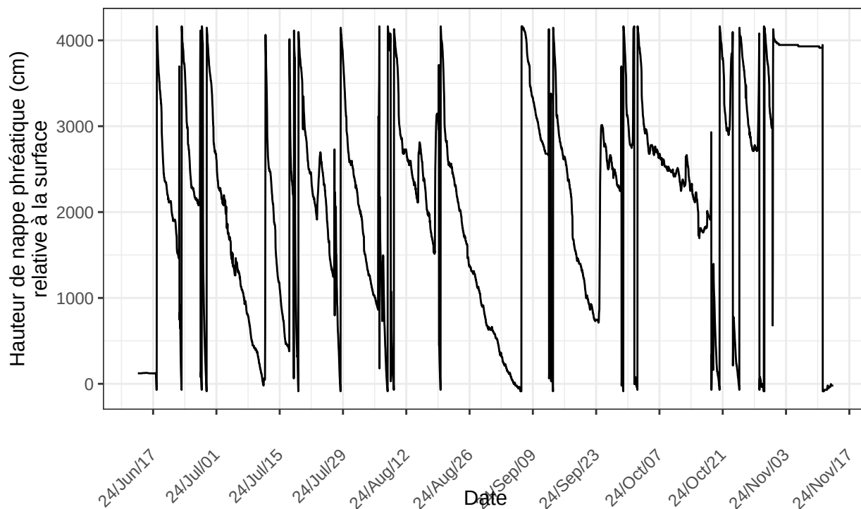
St-Henri, sonde no 42564 à l'emplacement STH.D2.p9m.2025 nombre de ligne du fichier : 4985
