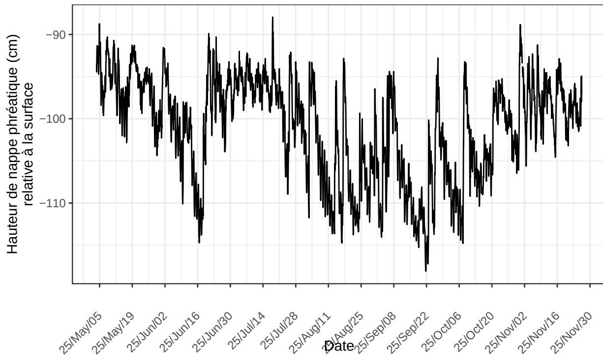
St-Henri, sonde no 22220787 à l'emplacement STH.D2.m1m.2025.bis nombre de ligne du fichier : 4986
