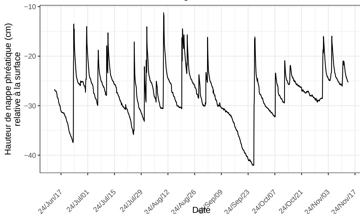
St-Henri, sonde no 41379 à l'emplacement STH.D2.p10,5m.2025 nombre de ligne du fichier : 4985
