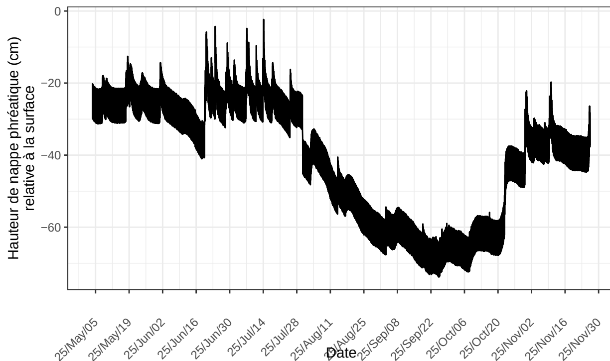
St-Henri, sonde no 41374 à l'emplacement STH.D2.p15m.2025 nombre de ligne du fichier : 4985
