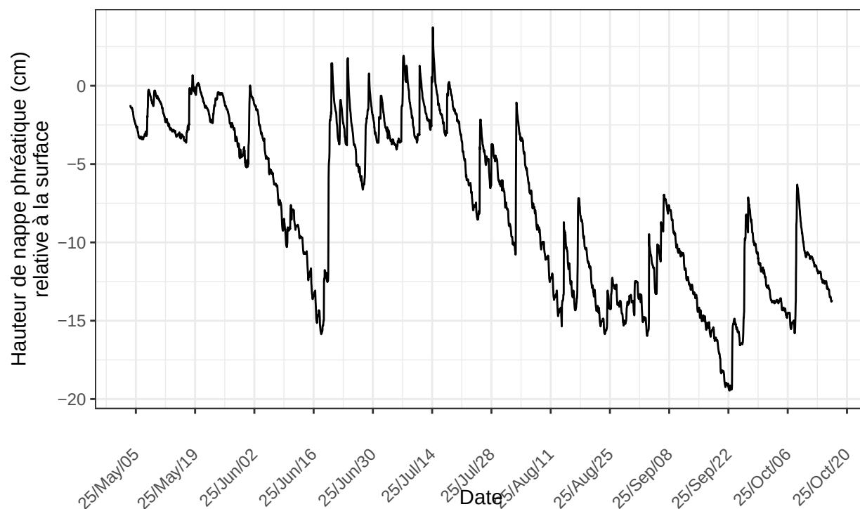
St-Henri, sonde no 41370 à l'emplacement STH.D2.p2,5m.2025 nombre de ligne du fichier : 3979
