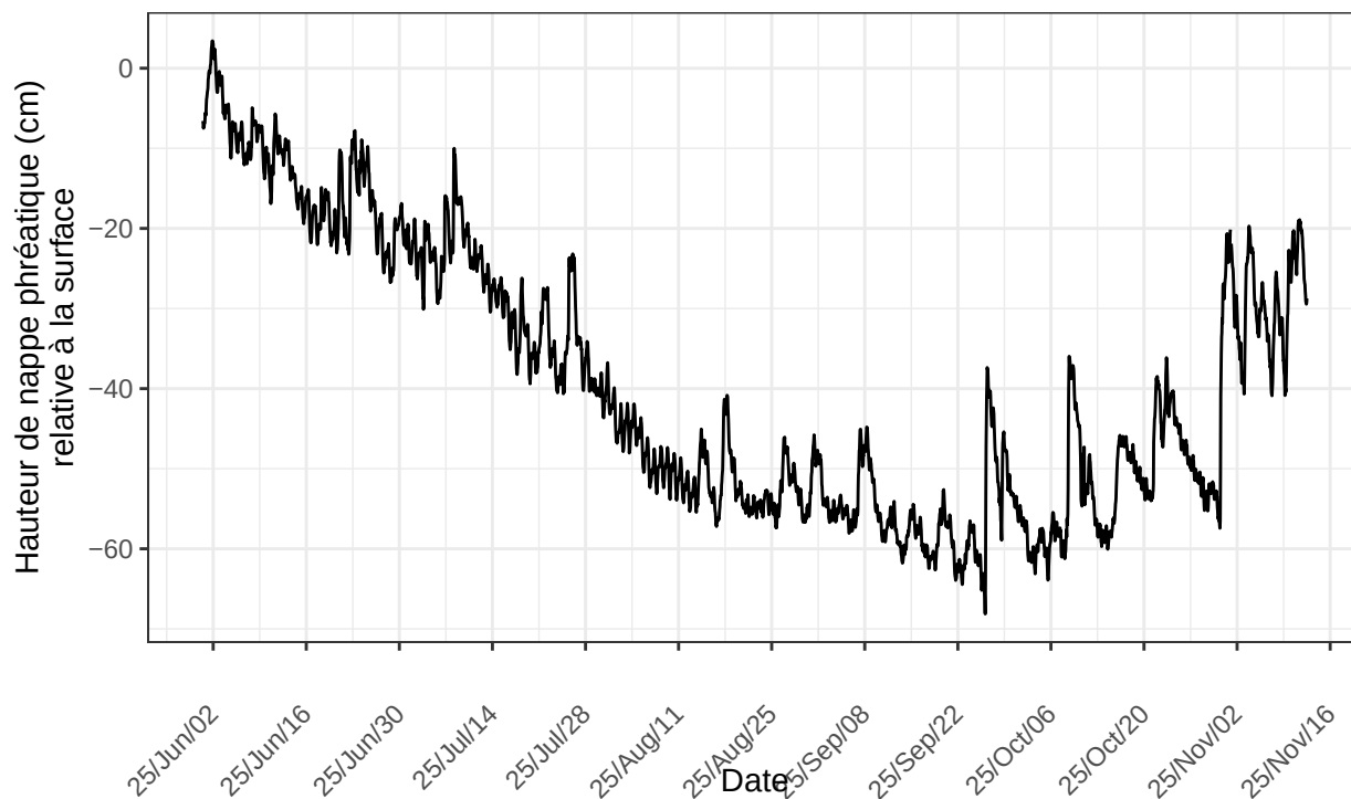
Inkerman, sonde no 22224403 à l'emplacement INK.Mare.D1.p7m.2025 nombre de ligne du fichier : 3985
