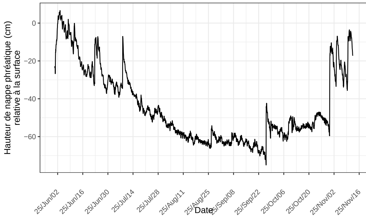
Inkerman, sonde no 22195244 à l'emplacement INK.ch3.C.1.2025 nombre de ligne du fichier : 1243
