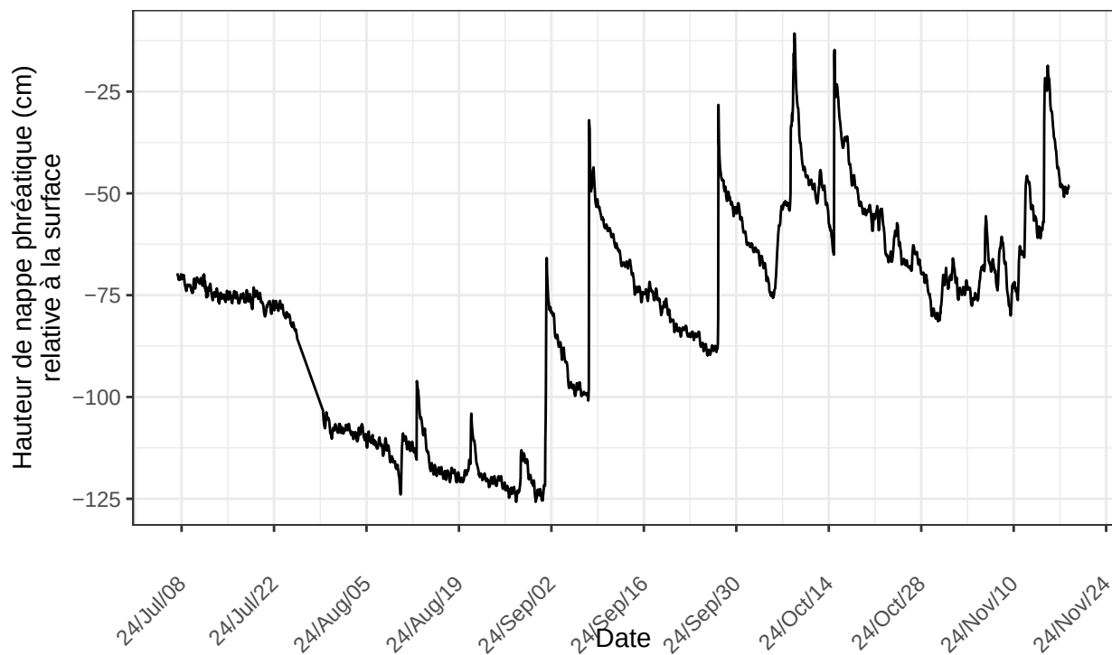
Inkerman, sonde no 20853328 à l'emplacement INK.EA.m4m.2024 nombre de ligne du fichier : 3148
