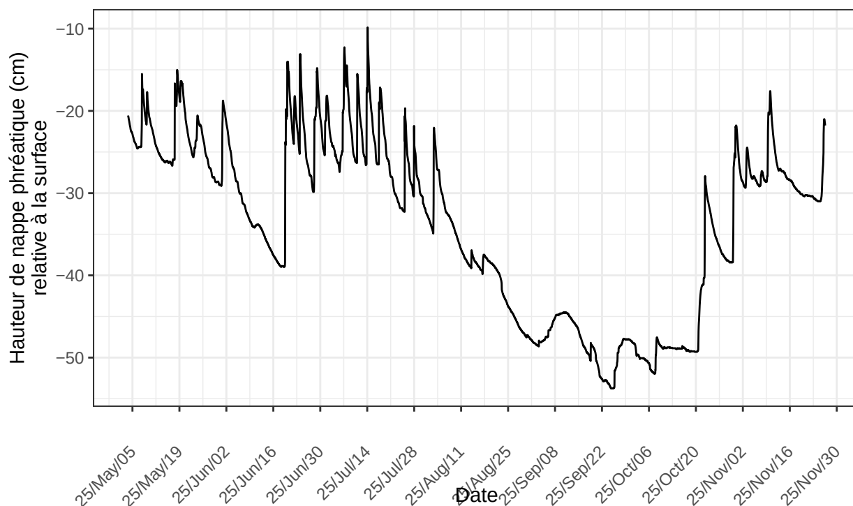
St-Henri, sonde no 41366 à l'emplacement STH.D3.30m.2024 nombre de ligne du fichier : 3692
