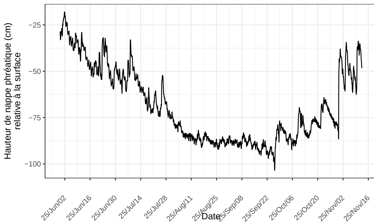
Inkerman, sonde no 22220791 à l'emplacement INK.Mare.A1.p7m.2025 nombre de ligne du fichier : 4011
