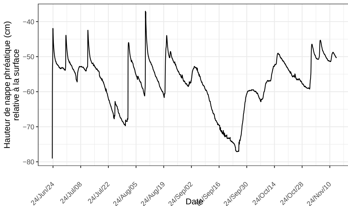
St-Henri, sonde no 42566 à l'emplacement STH.C.p6,75m.2025 nombre de ligne du fichier : 4989
