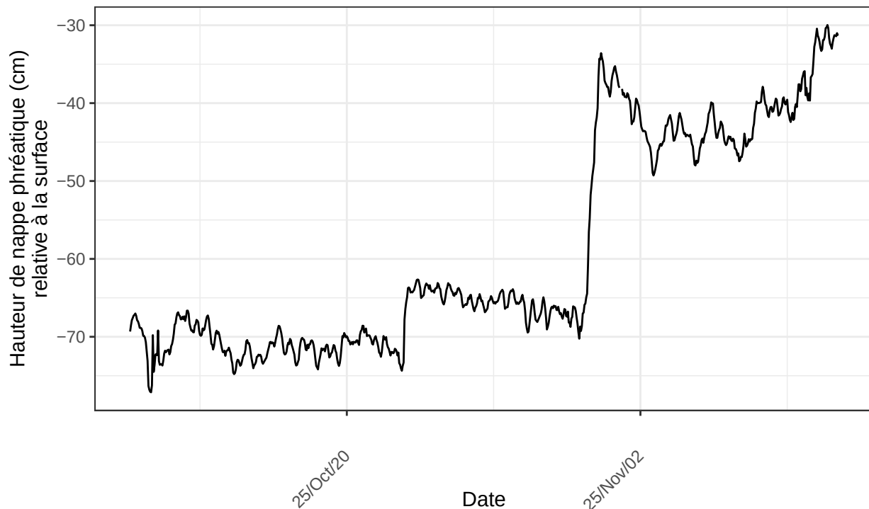
Inkerman, sonde no 22224397 à l'emplacement INK.Mare.D1.p14m.2025 nombre de ligne du fichier : 3985
