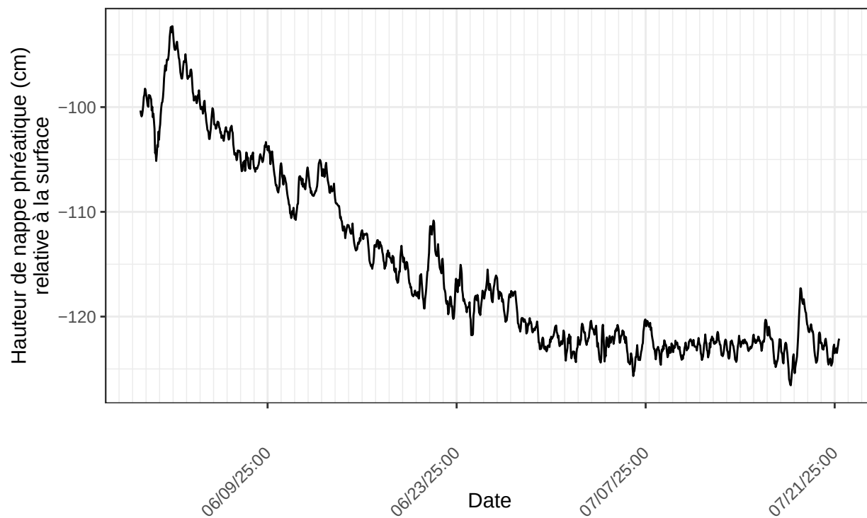
Inkerman, sonde no 22195244 à l'emplacement INK.ch3.C.1.2025 nombre de ligne du fichier : 1243
