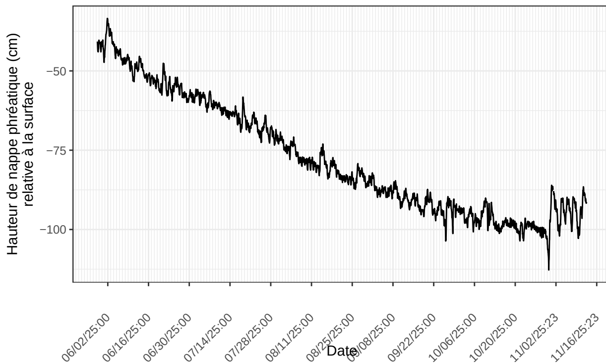
Inkerman, sonde no 22224390 à l'emplacement INK.Mare.D2.p30m.2025 nombre de ligne du fichier : 4034
