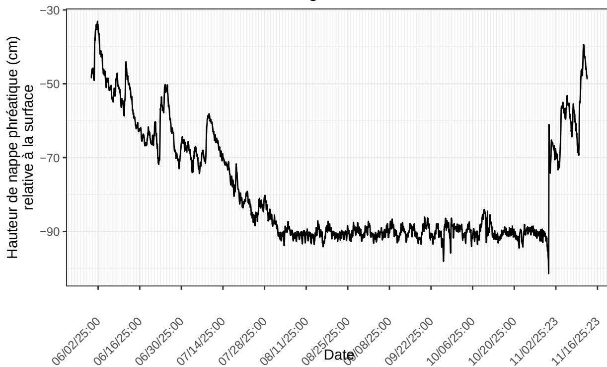
Inkerman, sonde no 22063138 à l'emplacement INK.ch3.berms.1.2025 nombre de ligne du fichier : 4006
