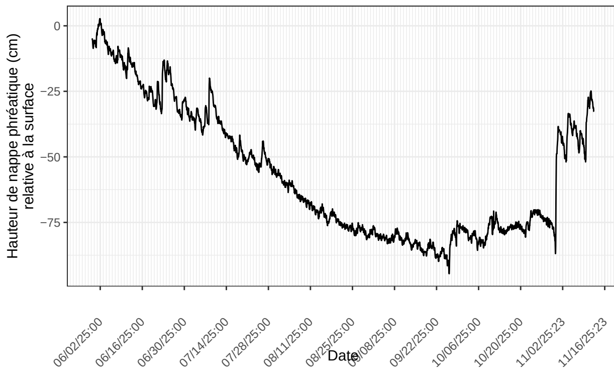
Inkerman", sonde no 22220785 à l'emplacement INK.pasMare.D2.p30m.2025 nombre de ligne du fichier : 4010
