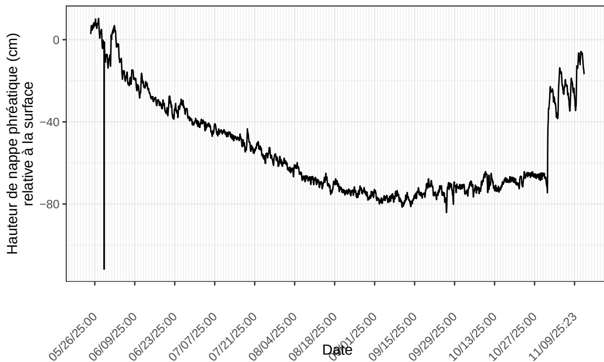
Inkerman", sonde no 22224392 à l'emplacement INK.pasMare.D2.m1m.2025 nombre de ligne du fichier : 4148
