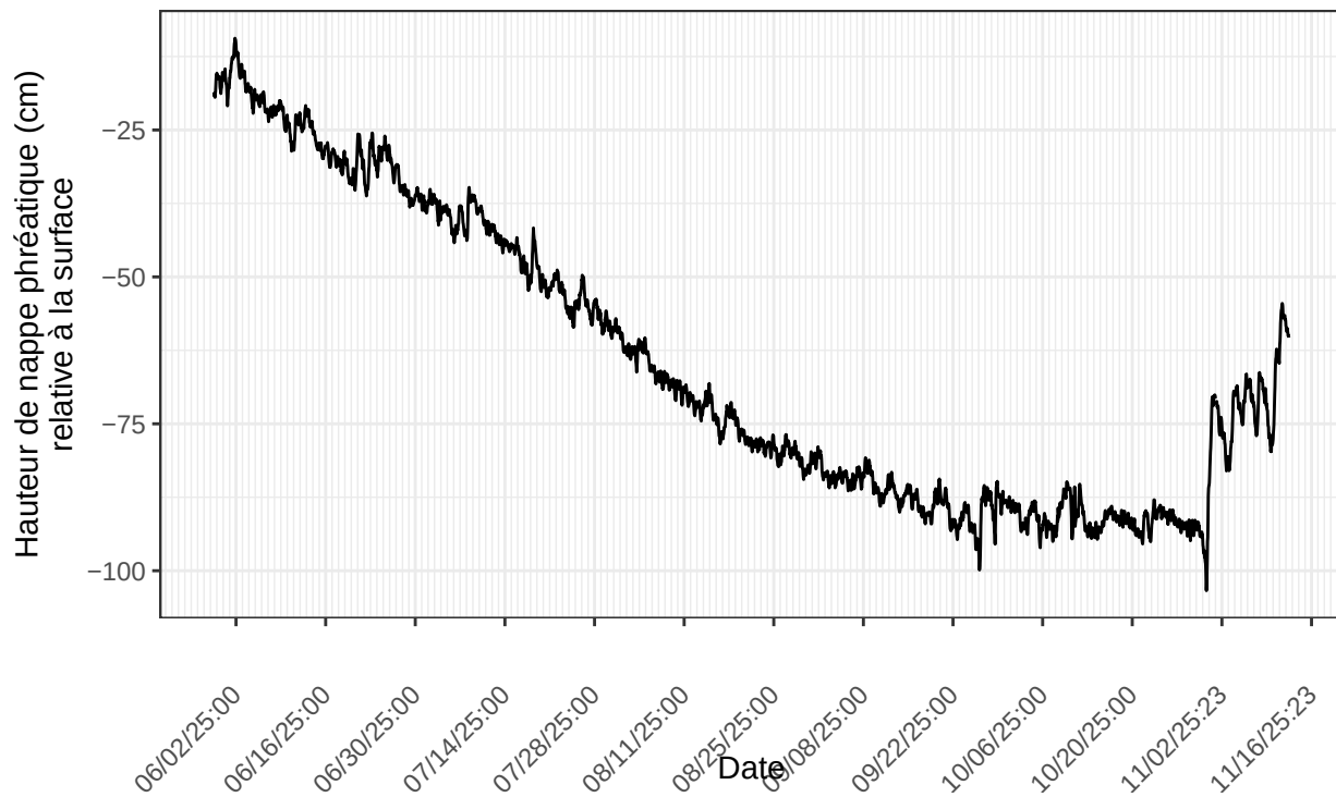
Inkerman, sonde no 22224394 à l'emplacement INK.pasMare.D1.p30m.2025 nombre de ligne du fichier : 4030
