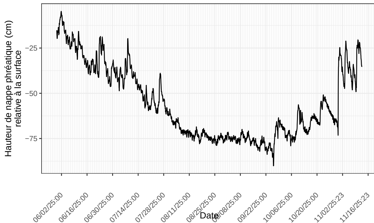
Inkerman, sonde no 22220791 à l'emplacement INK.Mare.A1.p7m.2025 nombre de ligne du fichier : 4012
