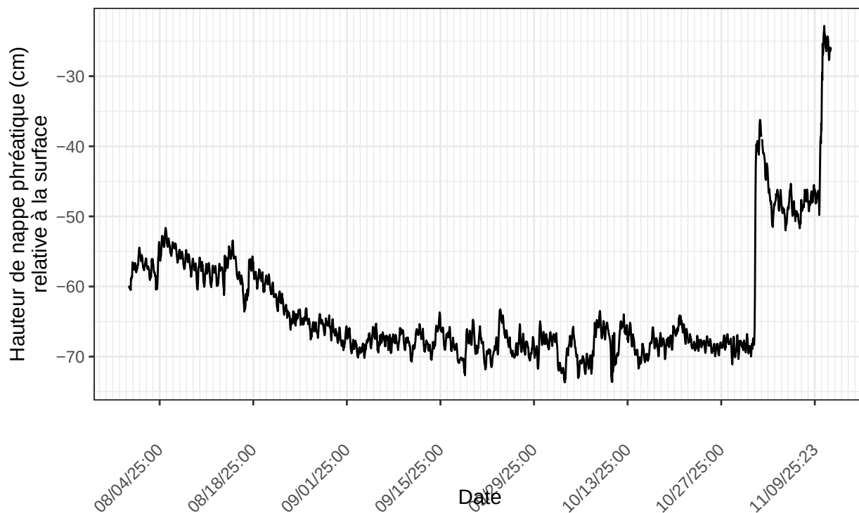
Inkerman", sonde no 22224414 à l'emplacement INK.pasMare.C2.p30m.2025 nombre de ligne du fichier : 4035
