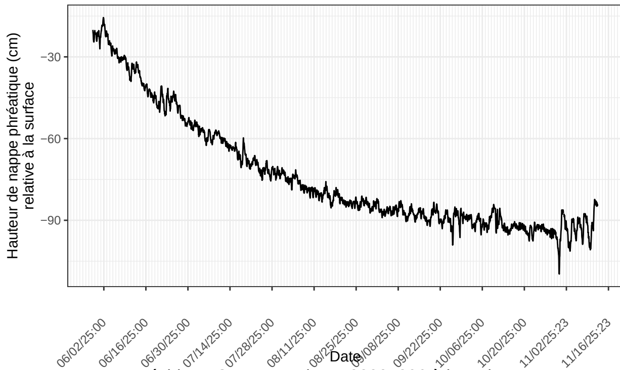
Président-Ouest, sonde no 22224396 à l'emplacement PRO.ch1.T3.chippd nombre de ligne du fichier : 810
