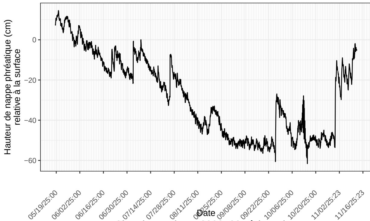
Burnt Church, sonde no 22224384 à l'emplacement BRNTC.ch1.C00.keptChannels.2025 nombre de ligne du fichier : 2783
