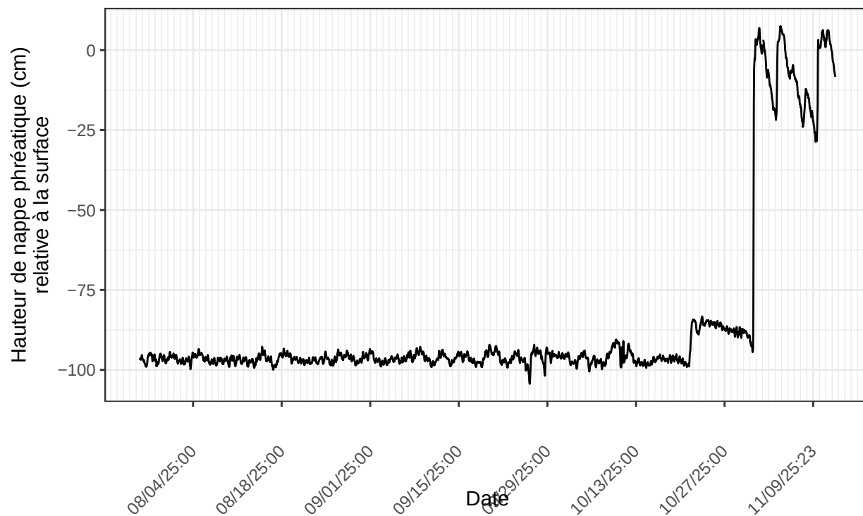
Inkerman", sonde no 22220789 à l'emplacement INK.ch3.rmvd.2.2025 nombre de ligne du fichier : 2638
