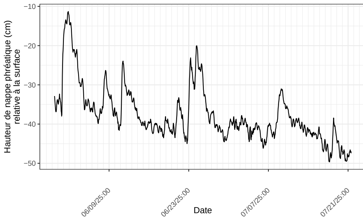
Président-Ouest, sonde no 22224386 à l'emplacement PRO.ch1.T1.gr.protec nombre de ligne du fichier : 1293
