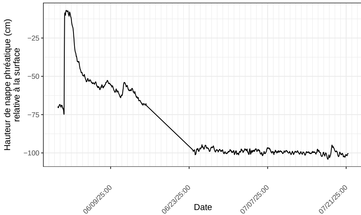
Inkerman, sonde no 22195248 à l'emplacement INK.ch3.C.3.2025 nombre de ligne du fichier : 1048
