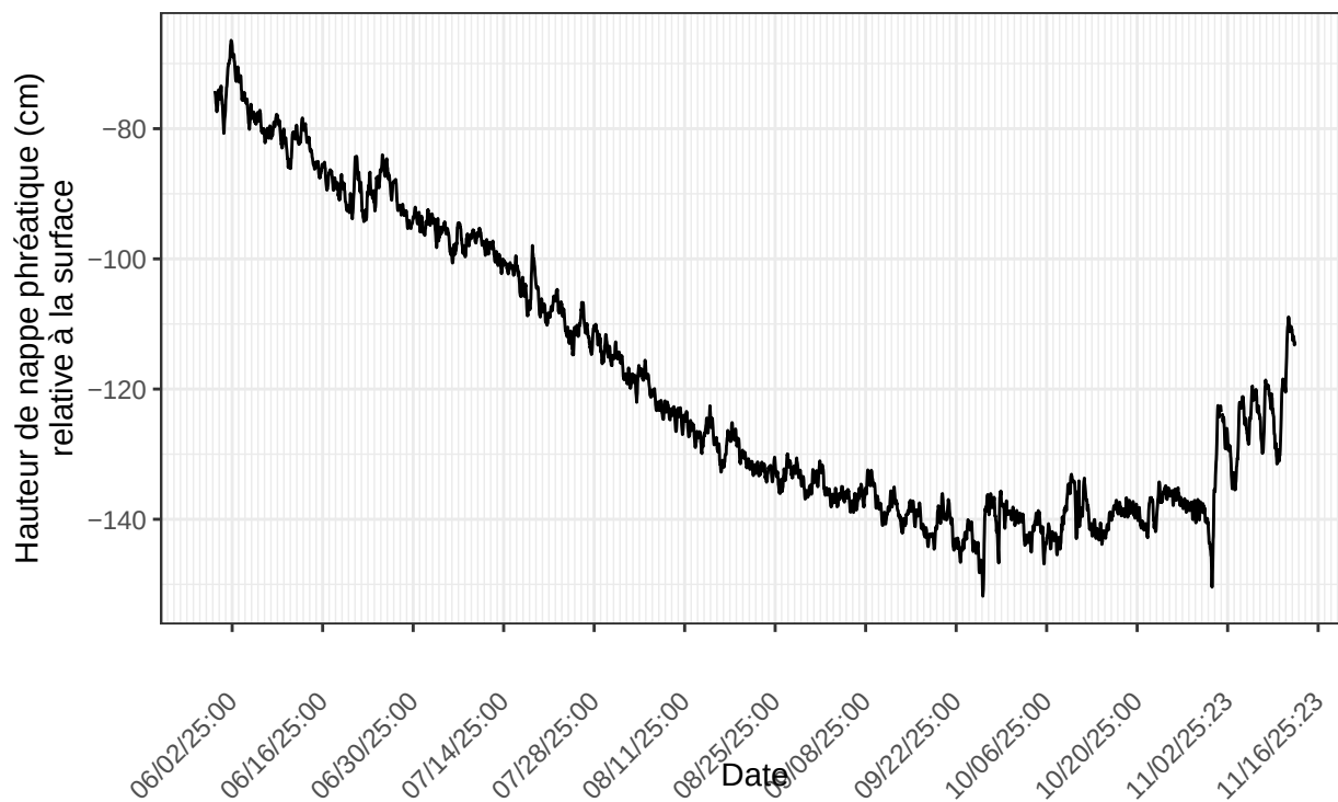
Inkerman", sonde no 22224388 à l'emplacement INK.pasMare.A1.p7m.2025 nombre de ligne du fichier : 4011
