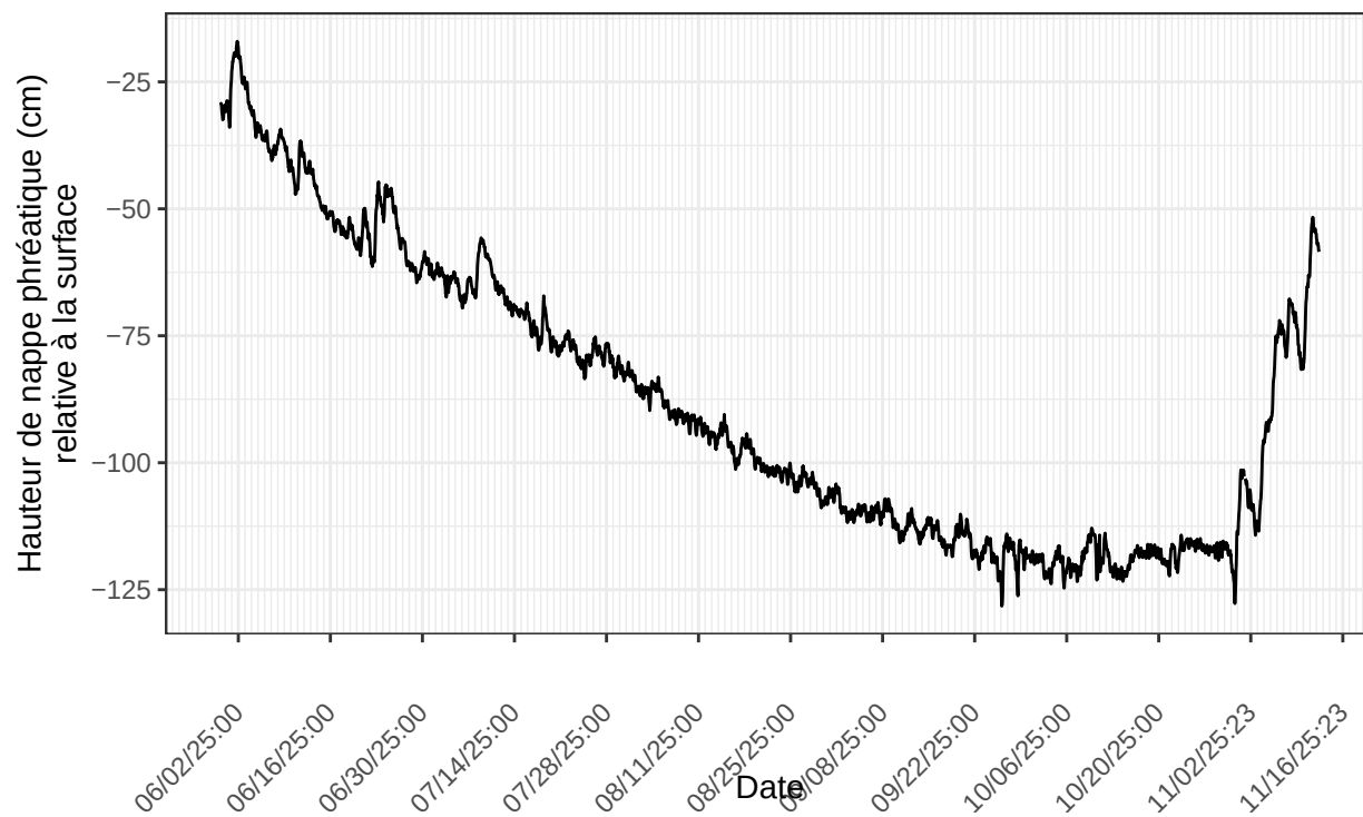
Inkerman, sonde no 22224409 à l'emplacement INK.pasMare.D2.p14m.2025 nombre de ligne du fichier : 4010
