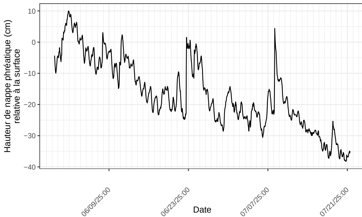
Inkerman, sonde no 22224413 à l'emplacement INK.Mare.A1.m1m.2025 nombre de ligne du fichier : 1252
