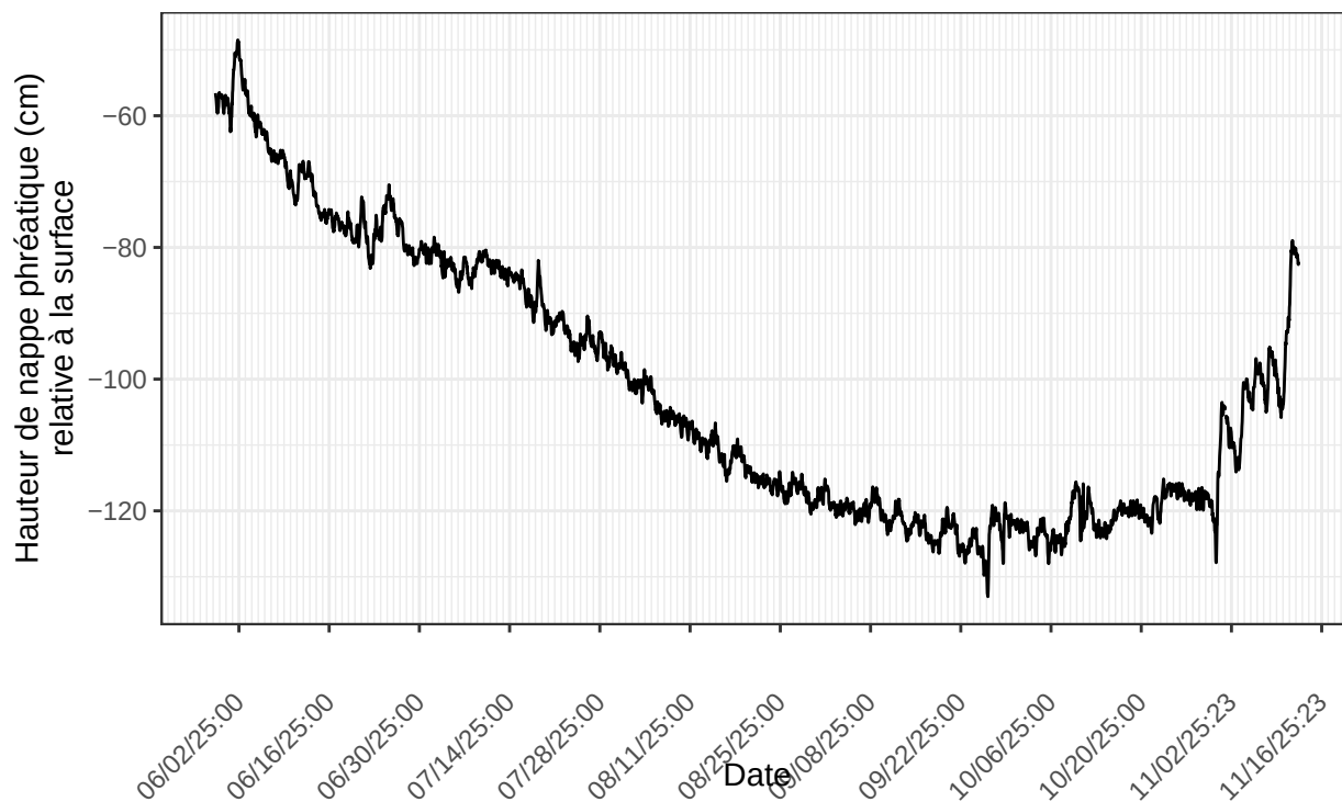
Inkerman, sonde no 22063139 à l'emplacement INK.Mare.A2.p14m.2025 nombre de ligne du fichier : 4034
