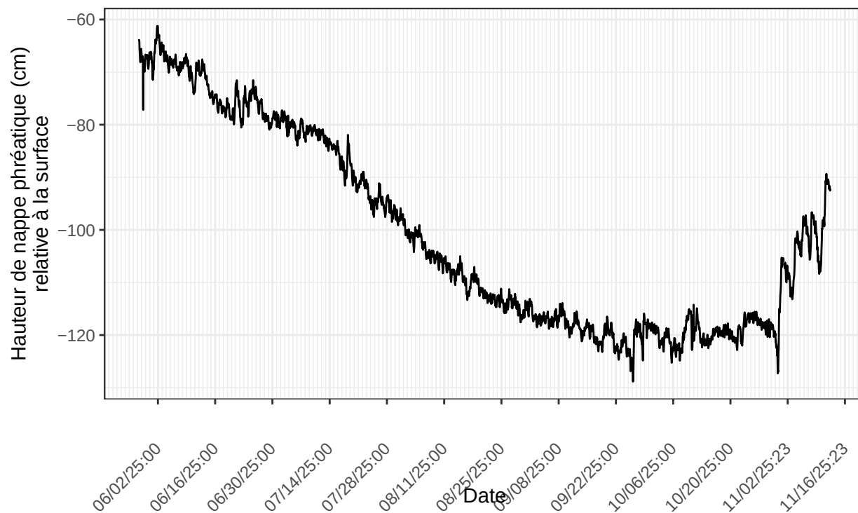
Inkerman", sonde no 22195242 à l'emplacement INK.pasMare.D1.p14m.2025 nombre de ligne du fichier : 4058
