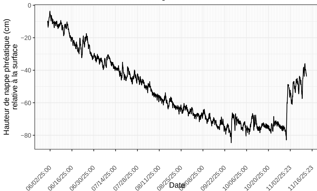
Burnt Church", sonde no 22224402 à l'emplacement BRNTC.ch1.T2.refrsh nombre de ligne du fichier : 2636
