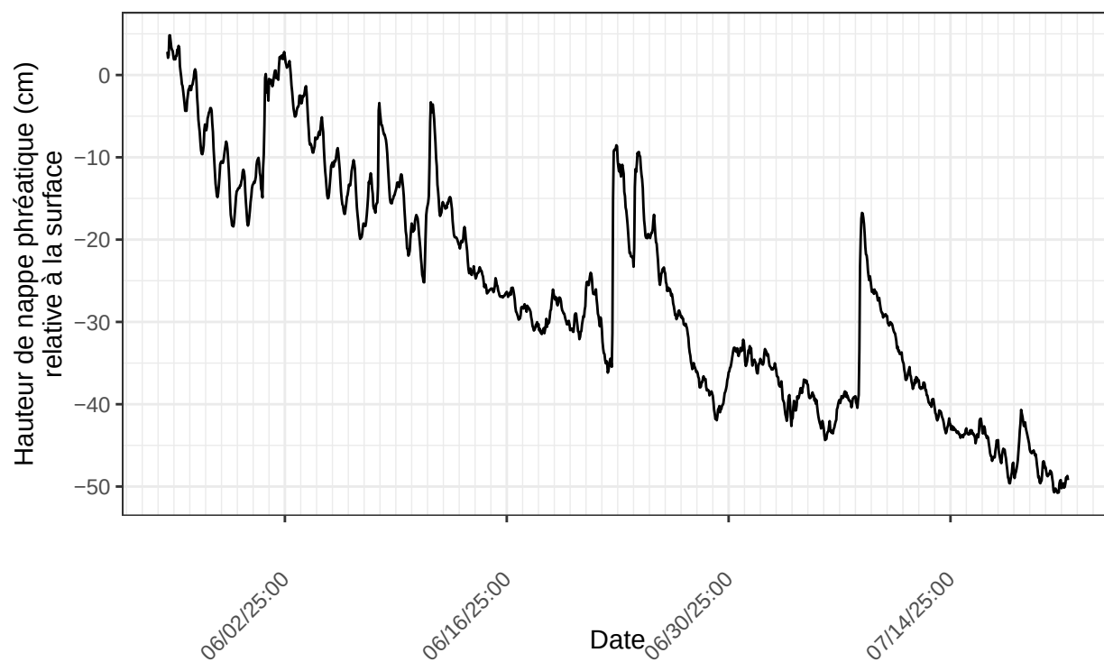
Inkerman, sonde no 22195241 à l'emplacement INK.pasMare.D1.m1m.2025 nombre de ligne du fichier : 1365
