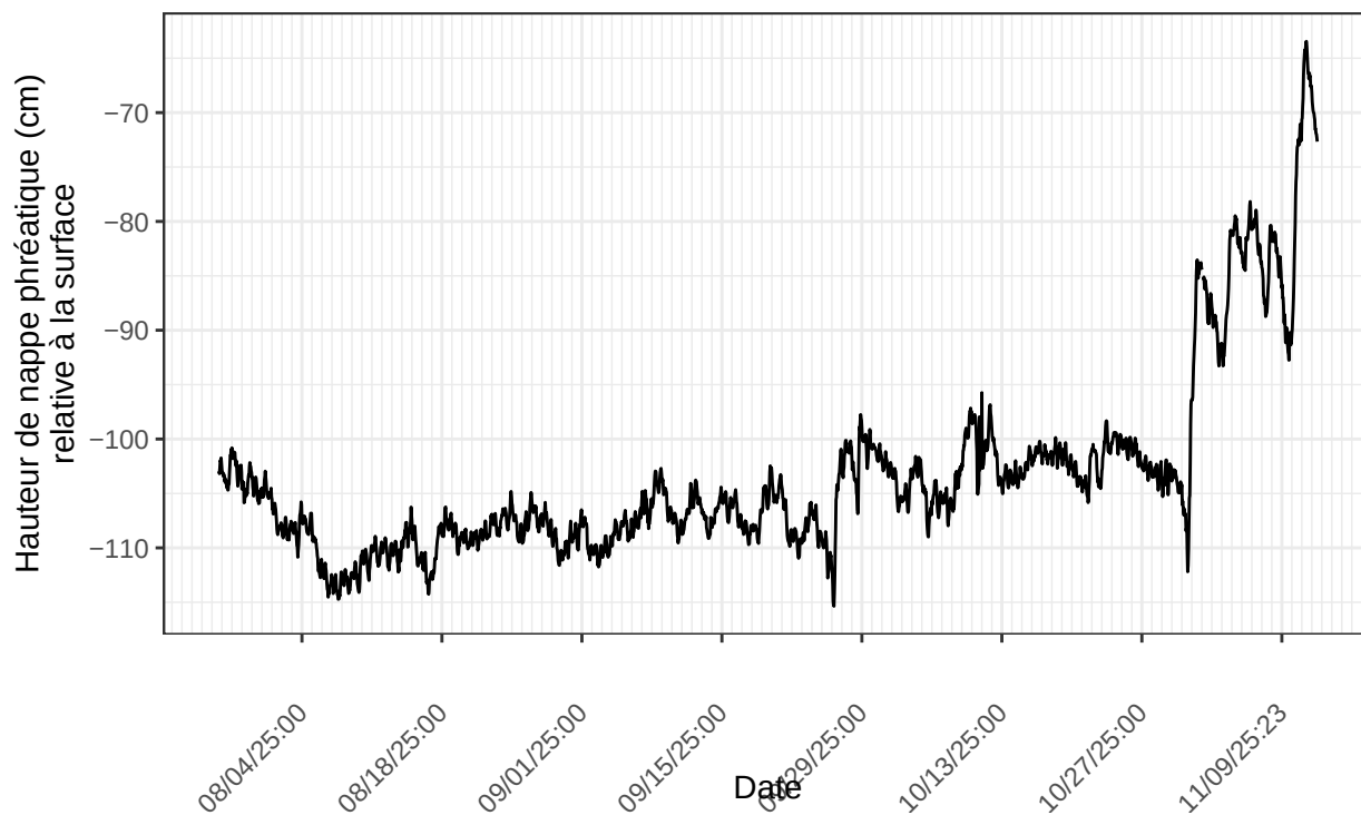
Inkerman", sonde no 22195246 à l'emplacement INK.ch3.C.1.2025 nombre de ligne du fichier : 2637
