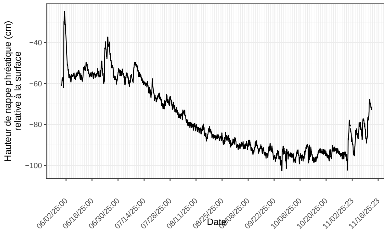
Inkerman", sonde no 22063159 à l'emplacement INK.pasMare.D2.p7m.2025 nombre de ligne du fichier : 4057
