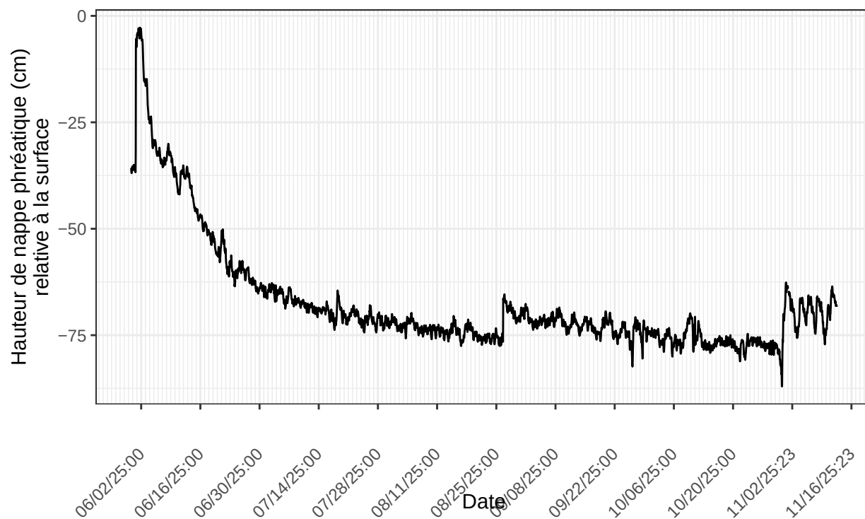
Inkerman", sonde no 22195245 à l'emplacement INK.ch3.berms.3.2025 nombre de ligne du fichier : 4006
