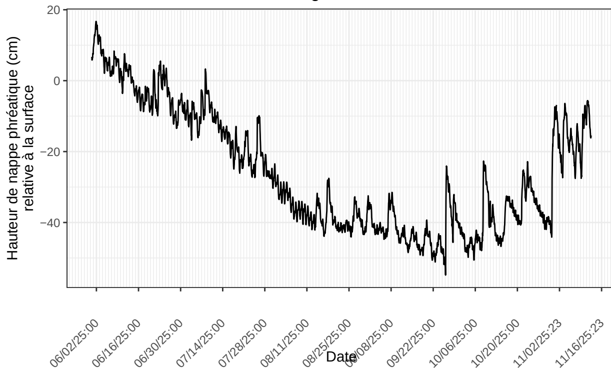
Président-Ouest, sonde no 22224407 à l'emplacement PRO.ch1.T2.refrsh nombre de ligne du fichier : 1293
