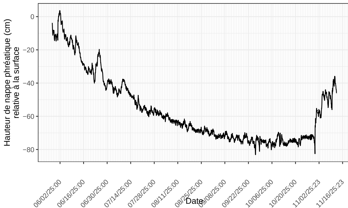
Inkerman, sonde no 22220784 à l'emplacement INK.pasMare.D1.p7m.2025 nombre de ligne du fichier : 4058
