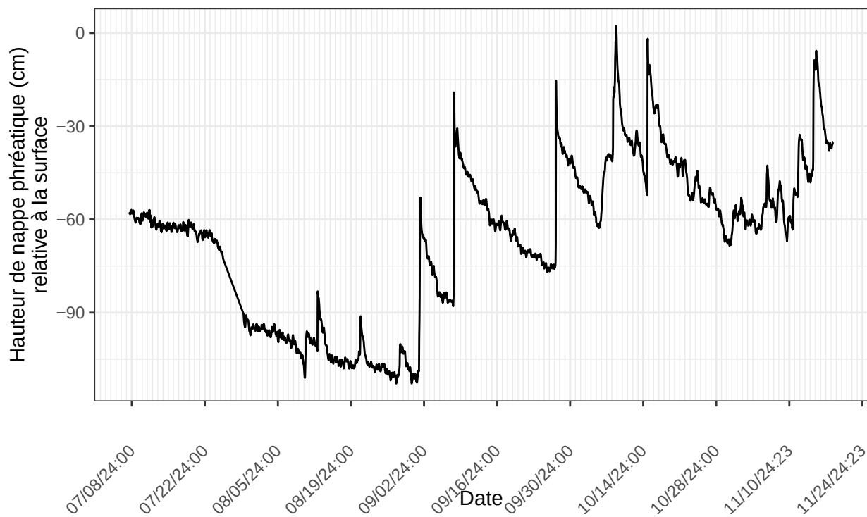
Inkerman, sonde no 20853328 à l'emplacement INK.EA.m4m.2024 nombre de ligne du fichier : 3144
