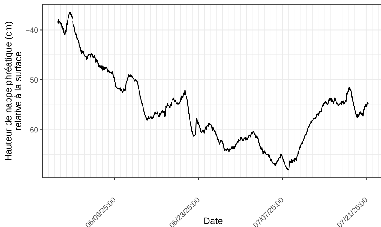
Titre De Tracé : Inkerman, sonde no 22224386 à l'emplacement INK.Mare.A2.m1m.2025 nombre de ligne du fichier : 1252
