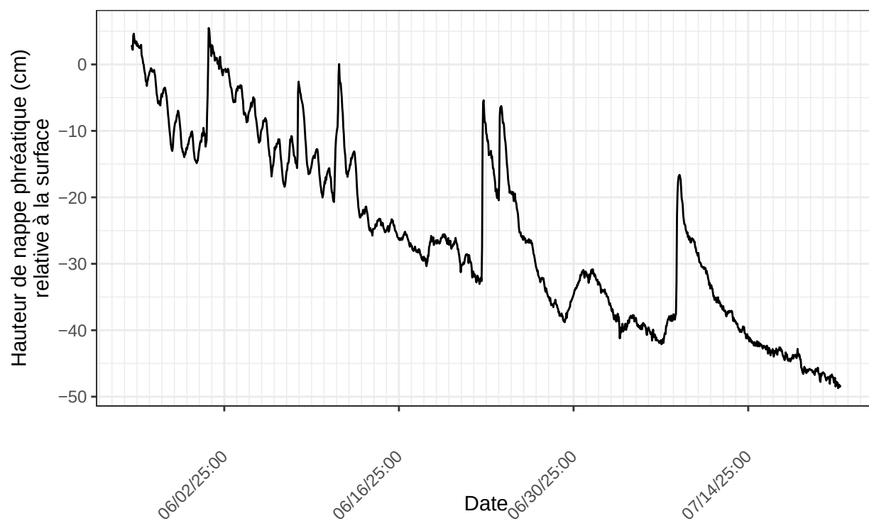
Titre De Tracé : Inkerman, sonde no 22195241 à l'emplacement INK.pasMare.D1.m1m.2025 nombre de ligne du fichier : 1365
