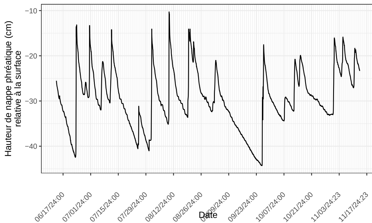
St-Henri, sonde no 42565 à l'emplacement STH.C.10m.2024 nombre de ligne du fichier : 3693
