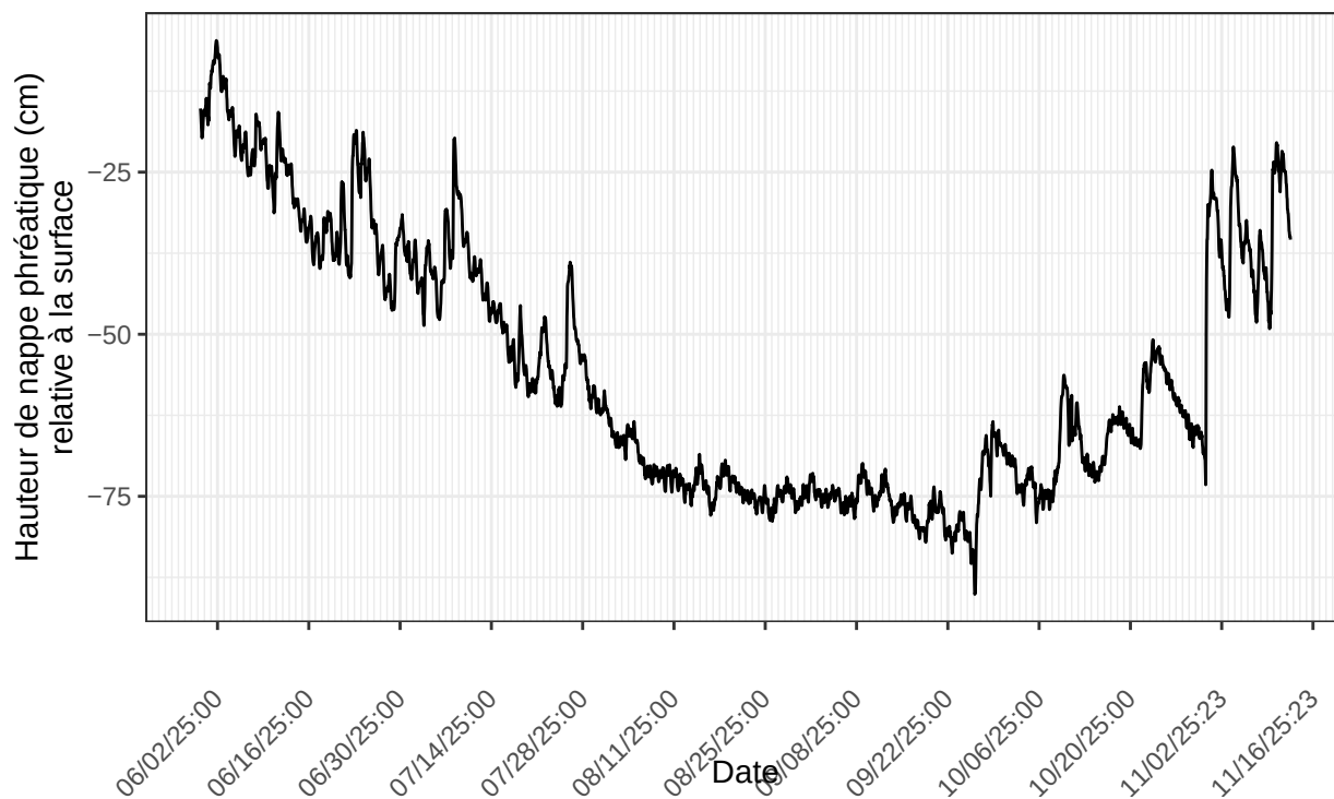
Titre De Tracé : Inkerman, sonde no 22220791 à l'emplacement INK.Mare.A1.p7m.2025 nombre de ligne du fichier : 4012
