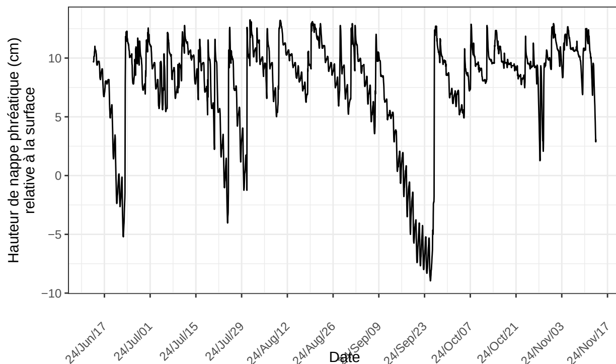
St-Henri, sonde no 42562 à l'emplacement STH.ch2.C.p7,75m.2025 nombre de ligne du fichier : 4988
