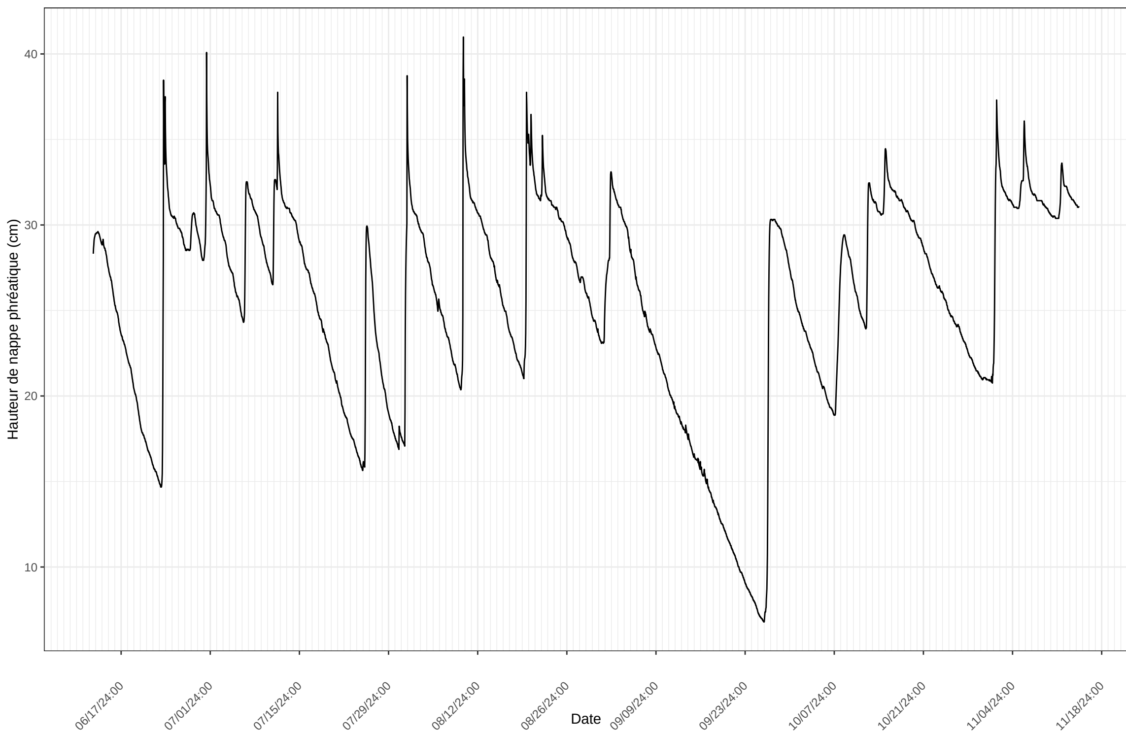
St-Henri, sonde no 41372 à l'emplacement A2.10m.2024
