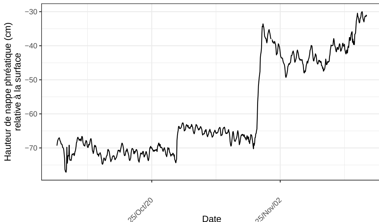
Inkerman, sonde no 22224397 à l'emplacement INK.ch2.MareD1.p14m.2025 nombre de ligne du fichier : 3985
