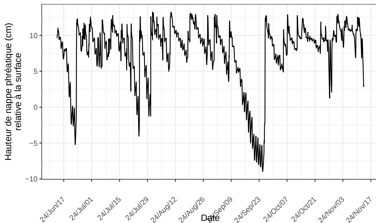
St-Henri, sonde no 41387 à l'emplacement STH.ch2.D3.m1m.2024 nombre de ligne du fichier : 3692
