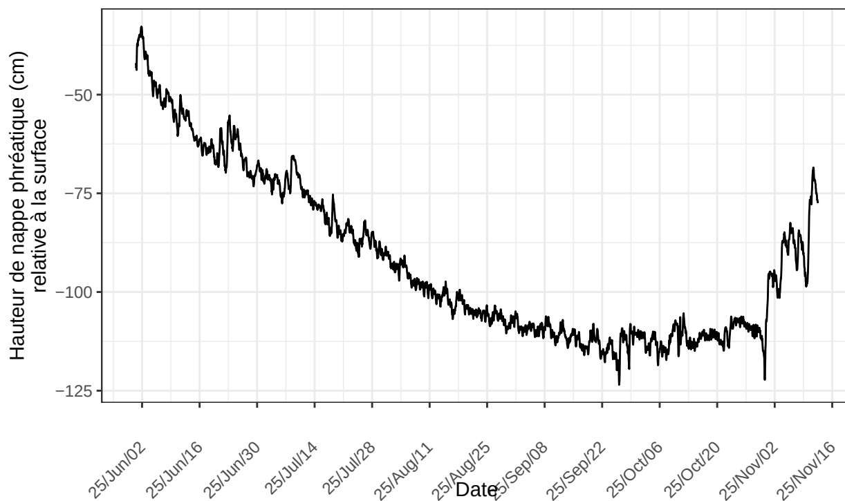
Inkerman, sonde no 22224397 à l'emplacement INK.ch2.MareD1.p14m.2025 nombre de ligne du fichier : 3985
