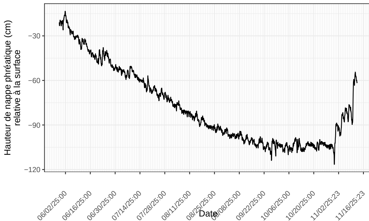
Titre De Tracé : Inkerman, sonde no 22224410 à l'emplacement INK.pasMare.A2.p30m.2025 nombre de ligne du fichier : 4031
