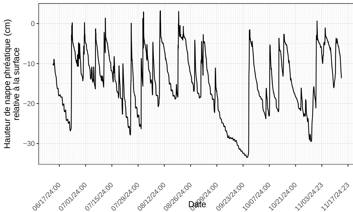
St-Henri, sonde no 41370 à l'emplacement STH.D3.7m.2024 nombre de ligne du fichier : 3693
