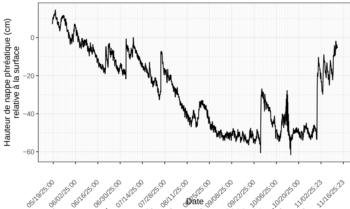
Titre De Tracé : Burnt Church, sonde no 22224384 à l'emplacement BRNTC.ch1.C00.keptChannels.2025 nombre de ligne du fichier : 2783
