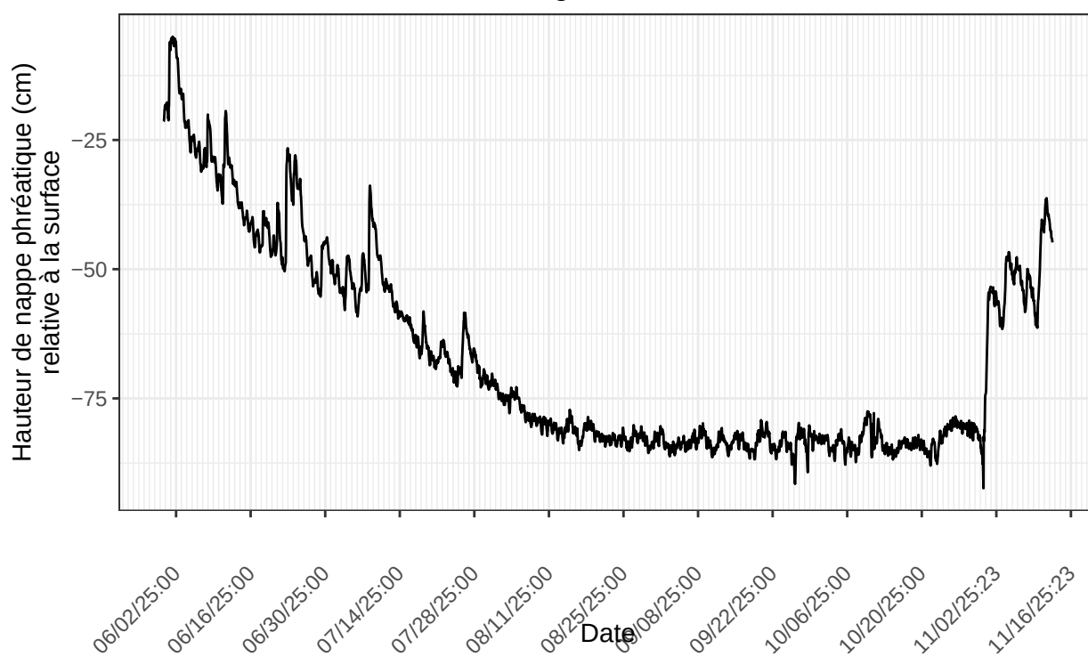
Titre De Tracé : Inkerman, sonde no 22063138 à l'emplacement INK.ch3.berms.1.2025 nombre de ligne du fichier : 4006
