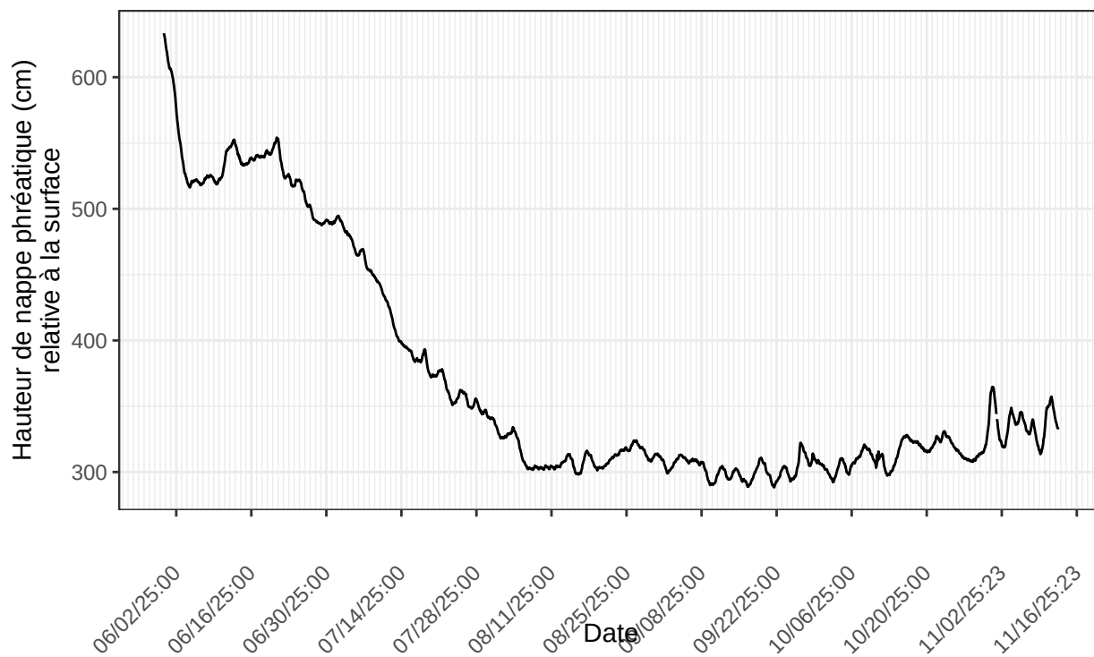
Titre De Tracé : Inkerman, sonde no 22220783 à l'emplacement INK.ch3.sprdd.3.2025 nombre de ligne du fichier : 4005
