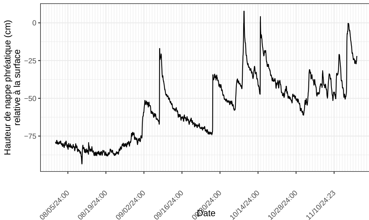
Titre De Tracé : Inkerman, sonde no 20853328 à l'emplacement INK.EA.m4m.2024 nombre de ligne du fichier : 3144
