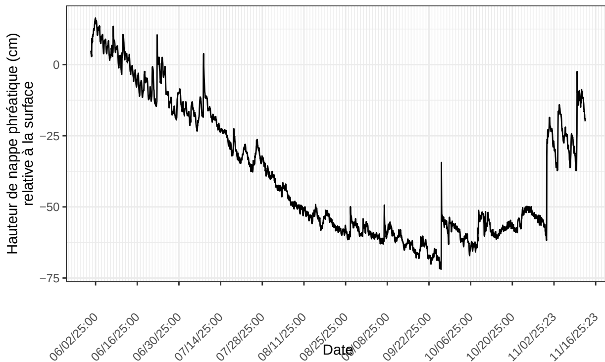
Titre De Tracé : Inkerman, sonde no 22063140 à l'emplacement INK.Mare.D2.p7m.2025 nombre de ligne du fichier : 3986
