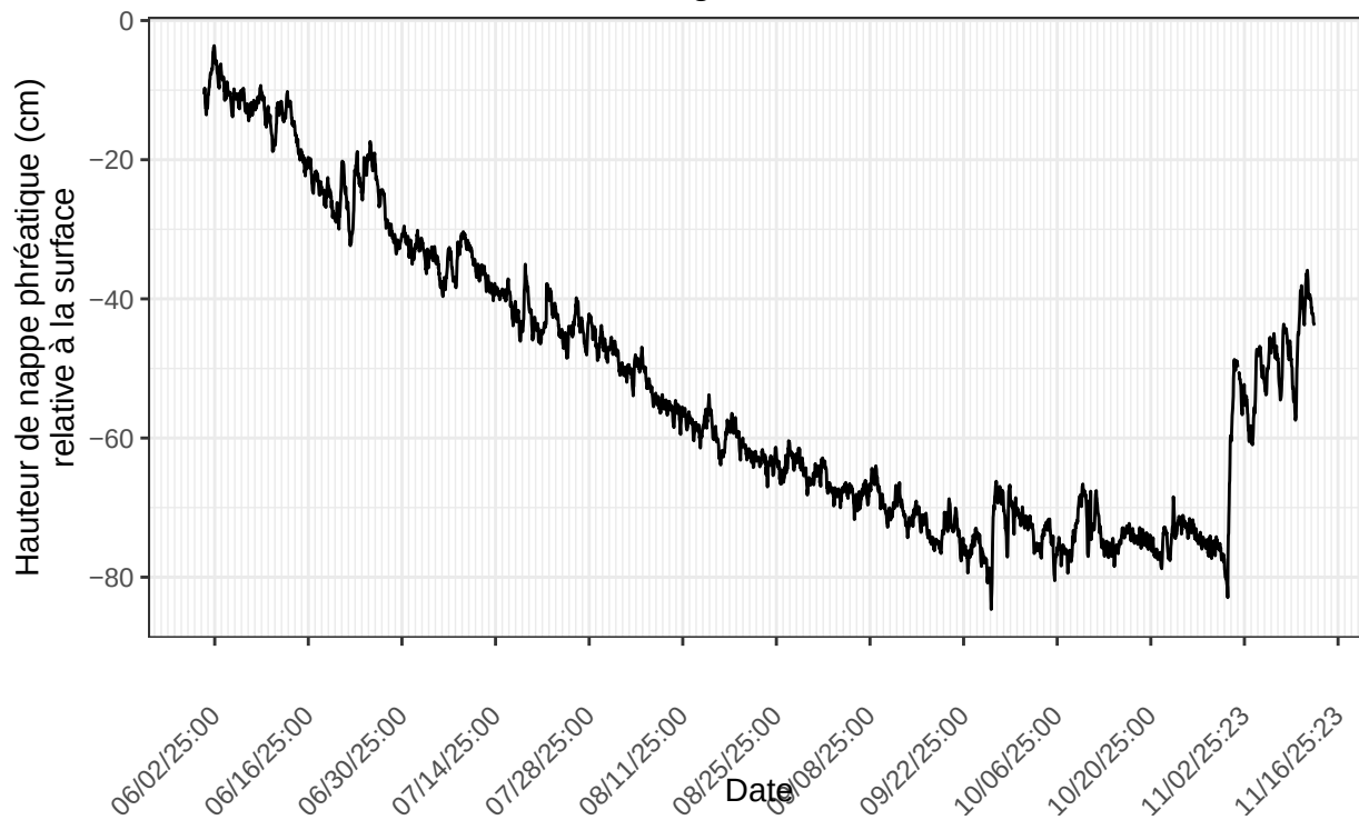
Inkerman, sonde no 22224400 à l'emplacement INK.Mare.D2.p14m.2025 nombre de ligne du fichier : 3986
