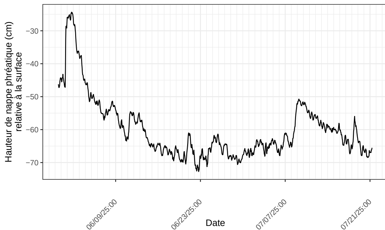
Inkerman, sonde no 22220788 à l'emplacement INK.ch3.rmvd.3.2025 nombre de ligne du fichier : 2638
