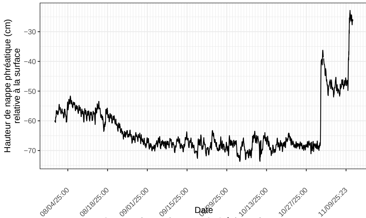
St-Henri, sonde no 41359 à l'emplacement STH.C.m1m.2024 nombre de ligne du fichier : 3669
