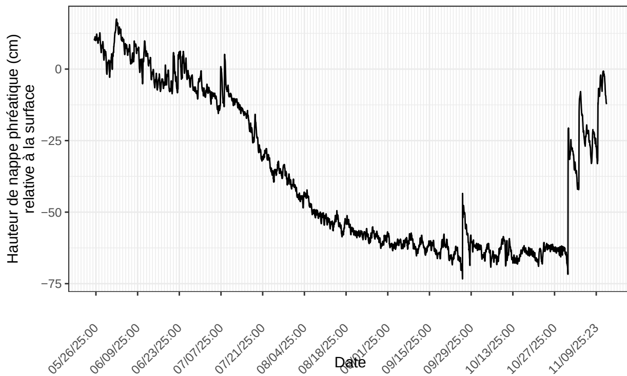
Inkerman", sonde no 22220786 à l'emplacement INK.pasMare.A2.m1m.2025 nombre de ligne du fichier : 4129
