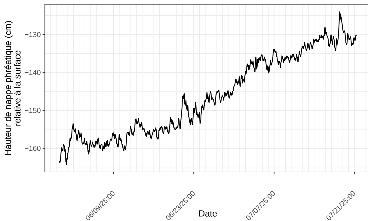
Inkerman, sonde no 22195246 à l'emplacement INK.ch3.C.2.2025 nombre de ligne du fichier : 1243
