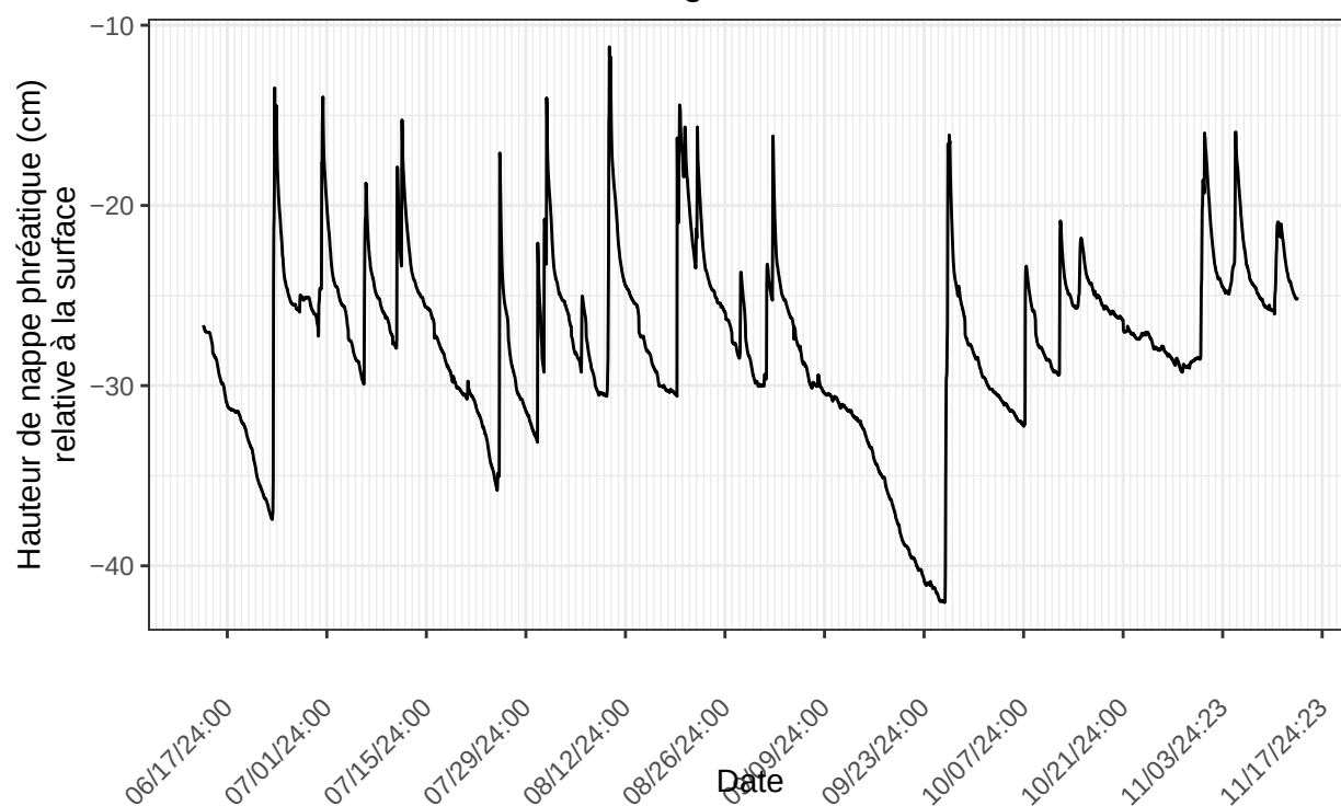
St-Henri, sonde no 41379 à l'emplacement STH.D2.p10,5m.2025 nombre de ligne du fichier : 0
