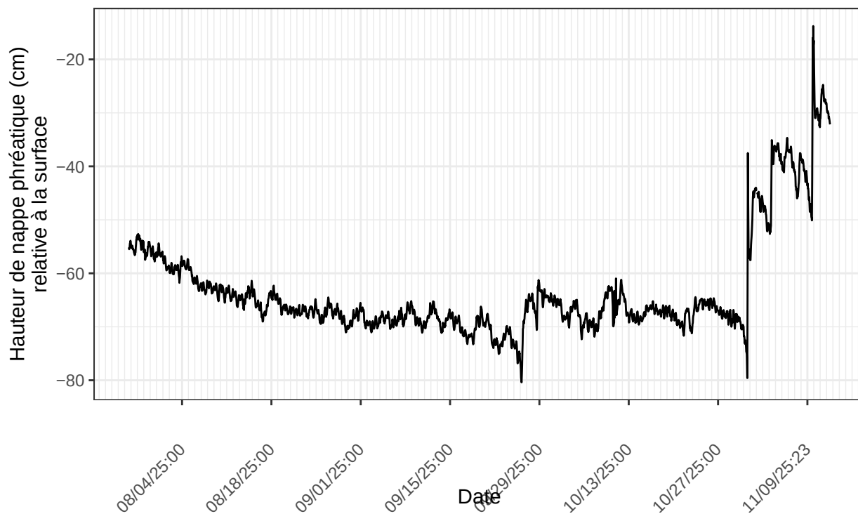
Inkerman", sonde no 22195248 à l'emplacement INK.ch3.C.3.2025 nombre de ligne du fichier : 2637
