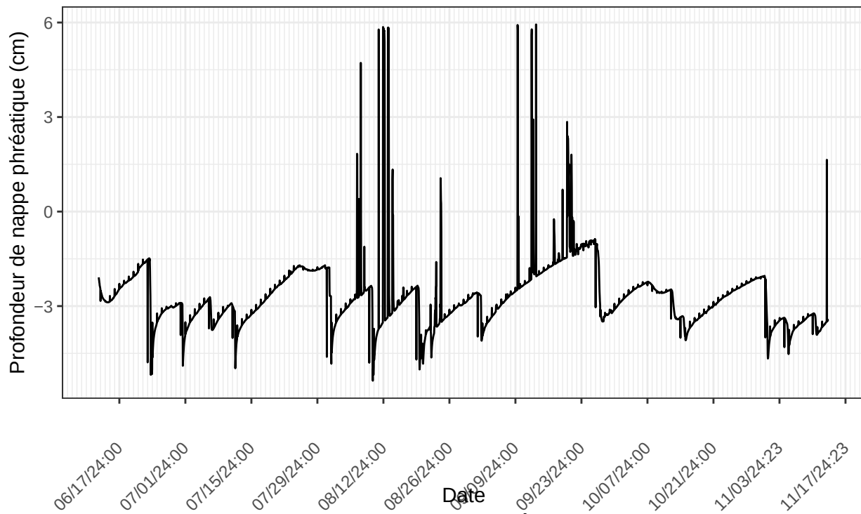
St-Henri, sonde no 41366 à l'emplacement D3.30m.2024 nombre de ligne du fichier : 3716
