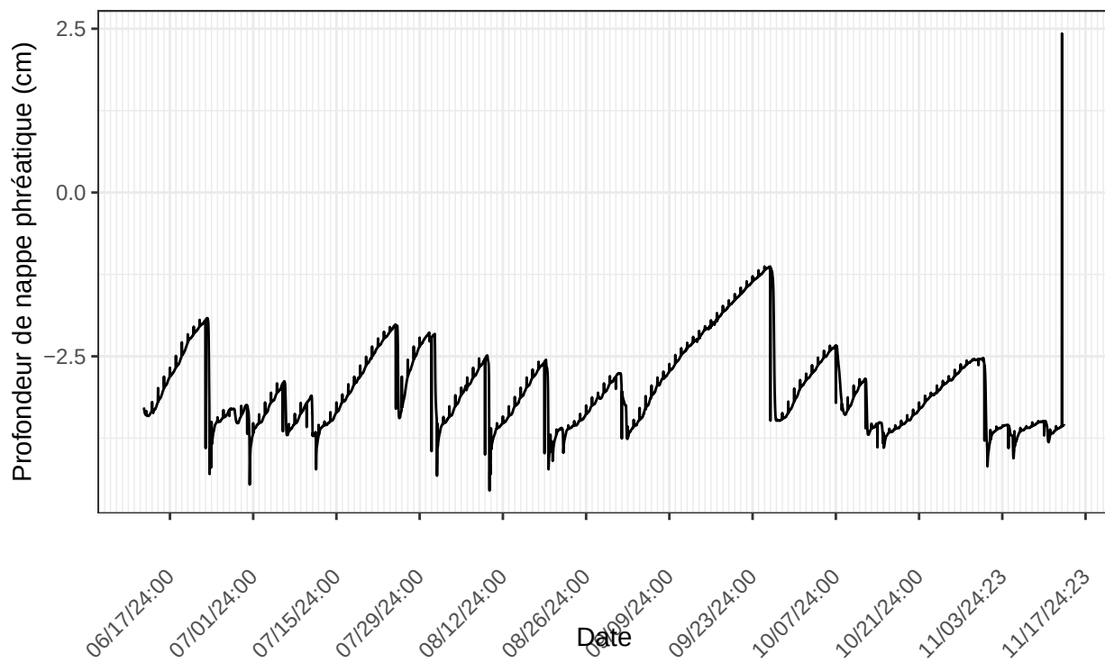
St-Henri, sonde no 41372 à l'emplacement A2.10m.2024 nombre de ligne du fichier : 3716
