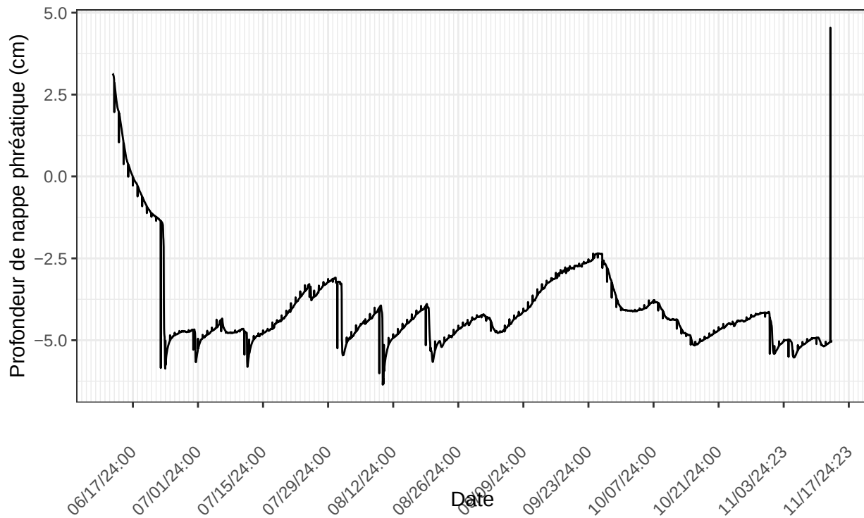
St-Henri, sonde no 42566 à l'emplacement C.7m.2024 nombre de ligne du fichier : 3716
