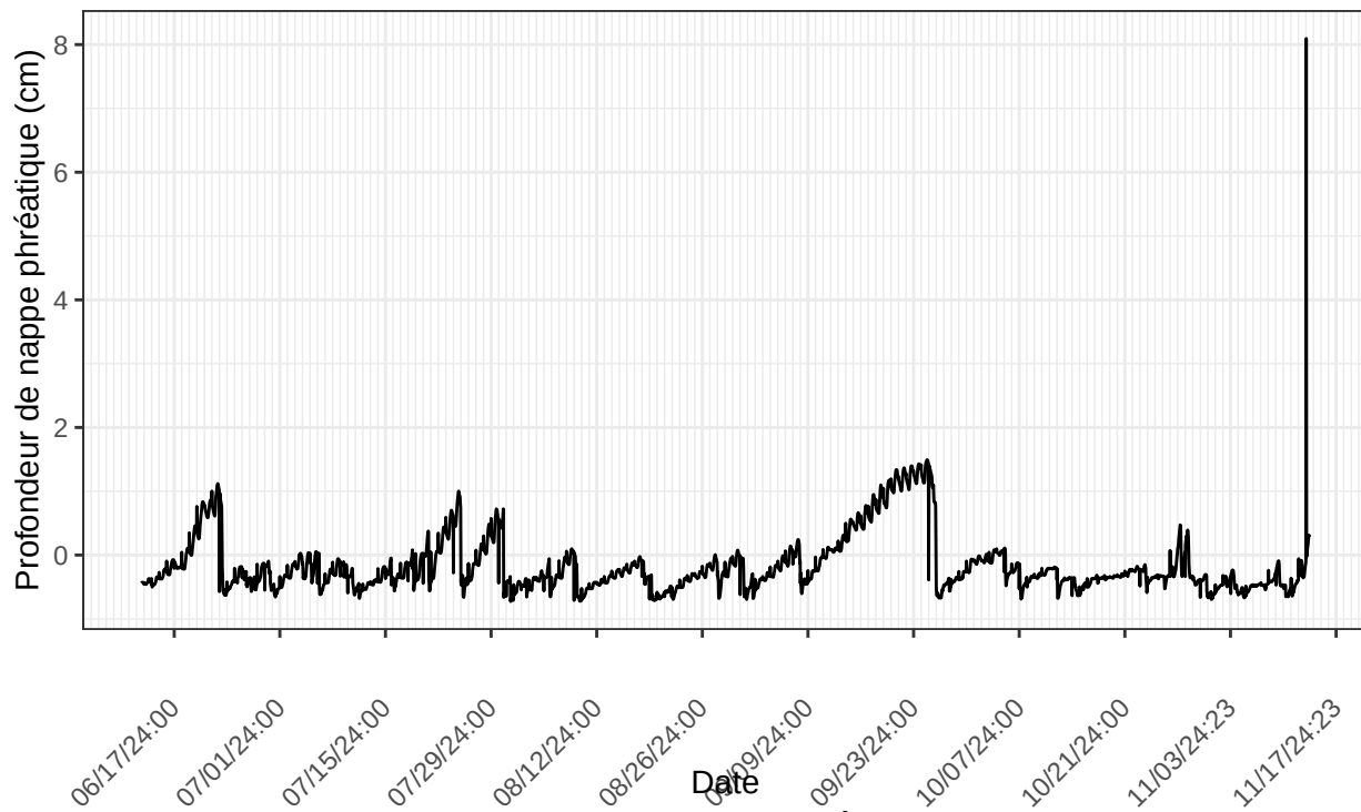
St-Henri, sonde no 42564 à l'emplacement C.30m.2024 nombre de ligne du fichier : 3716
