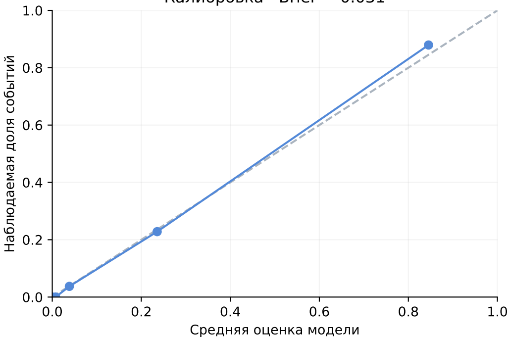
Калибровка · Brier = 0.031
