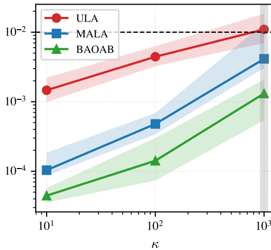
Anisotropic
