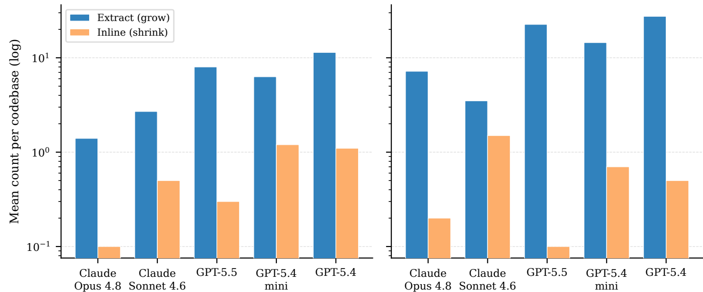
Algorithms (001-050) (n=50)
