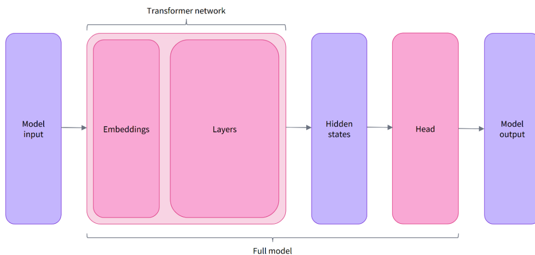
图 13.2 预训练模型精调的模型结构
