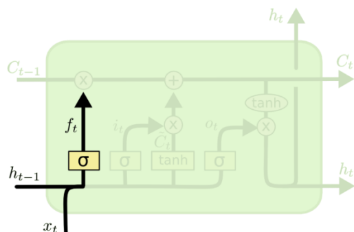
图 8.18 LSTM 块的第一层：一个 Sigmoid 层
