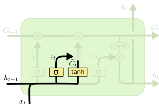
图 8.19 LSTM 块的第二，三层
