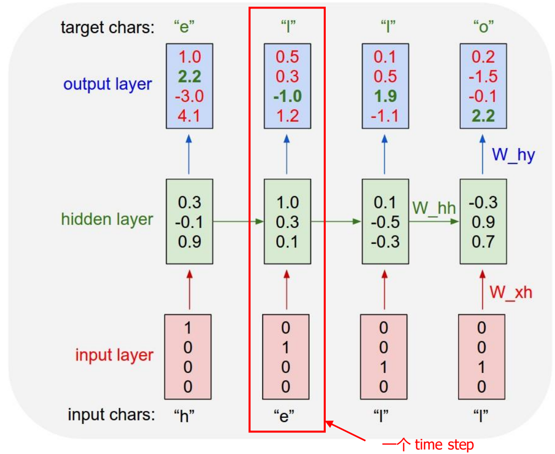
图 8.5 展开的 RNN 实例
